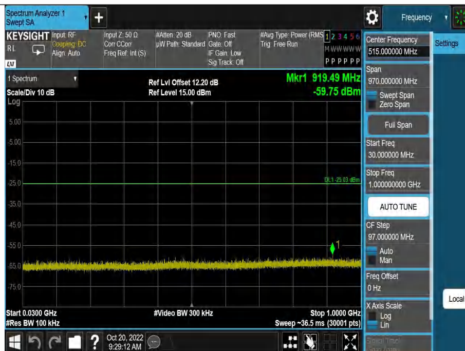
DH5-Ant1-2402-30~1000--5.03
