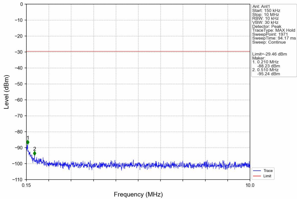
1_MCH_2441MHz_Ant1_NTNV
