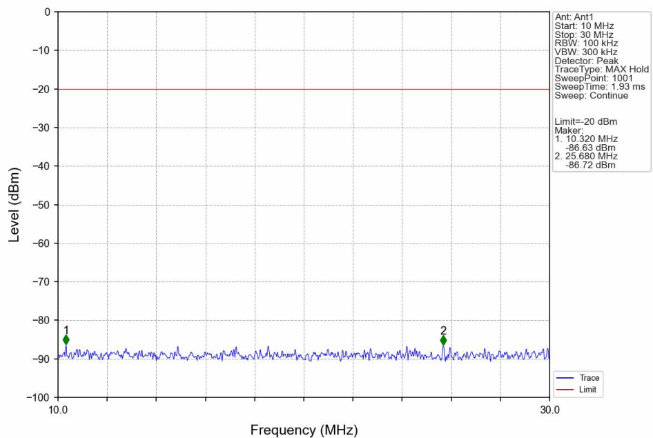
1_LCH_2402MHz_Ant1_NTNV
