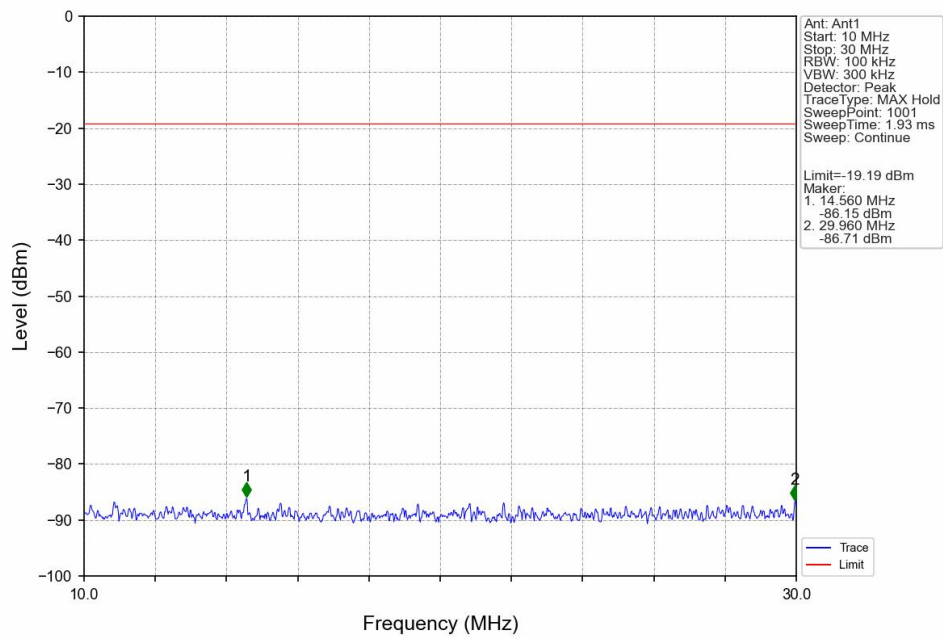
1_HCH_2480MHz_Ant1_NTNV
