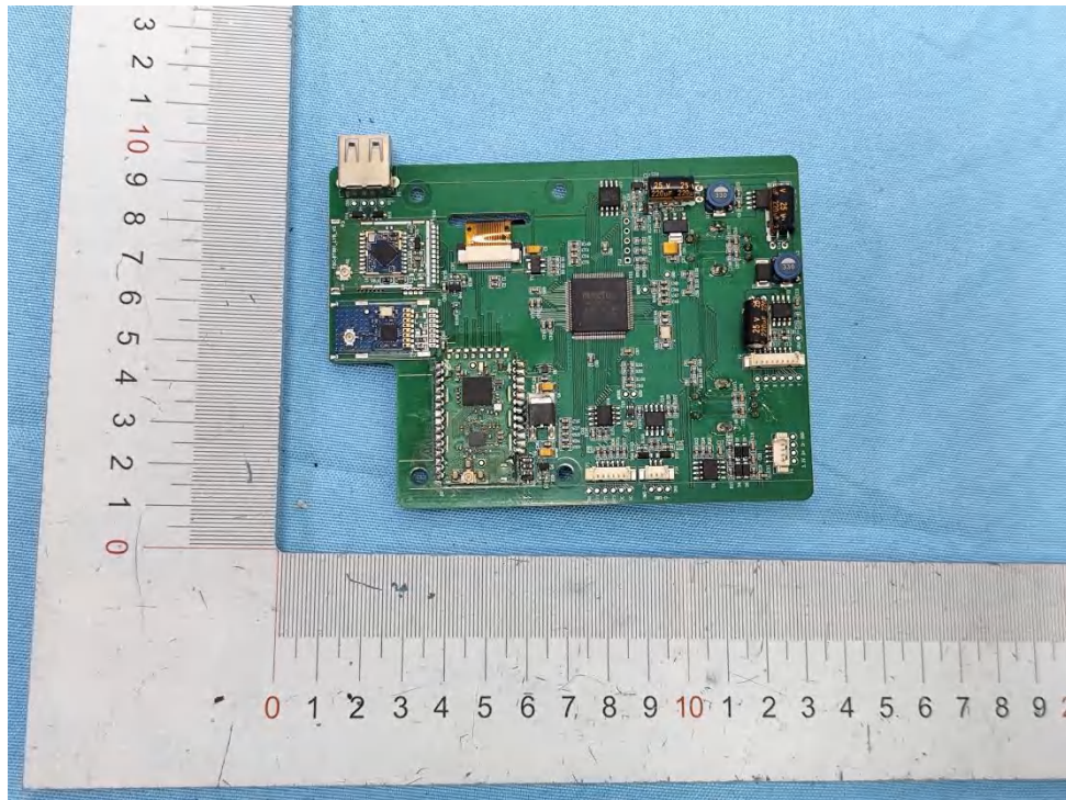
BLE Antenna Interface
