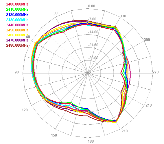
E2 Face
