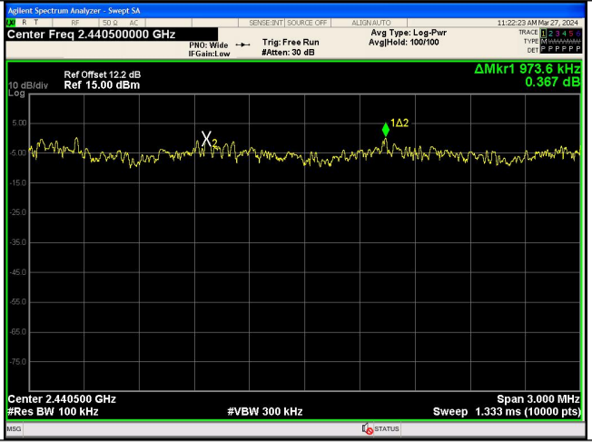
8DPSK
