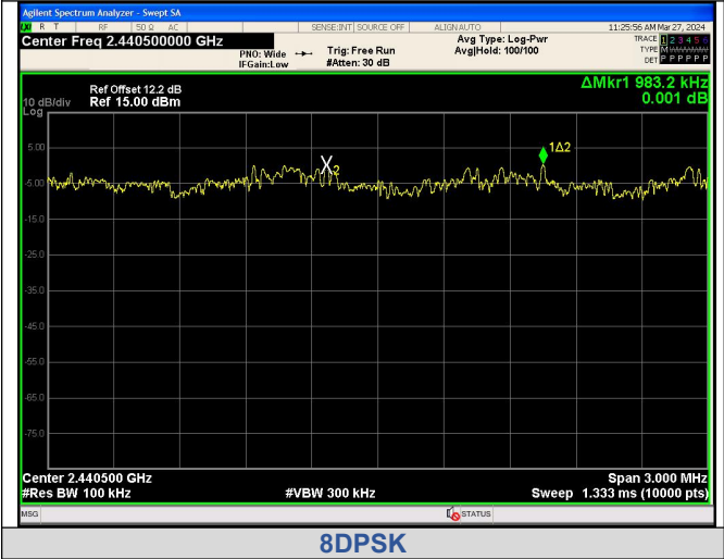
8DPSK
