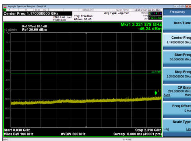
,Plot 3,30MHz~2310MHz-802.11g,2437MHz
