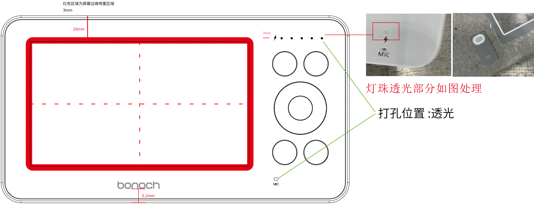
19*3.3mm 丝印颜色：银色 正视图
