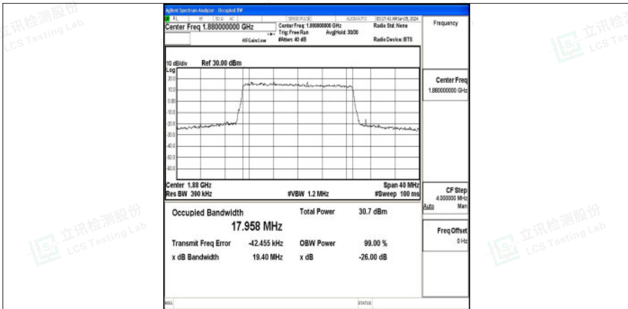
Band2-20MHz-QPSK-18900-100RB#0-PASS
