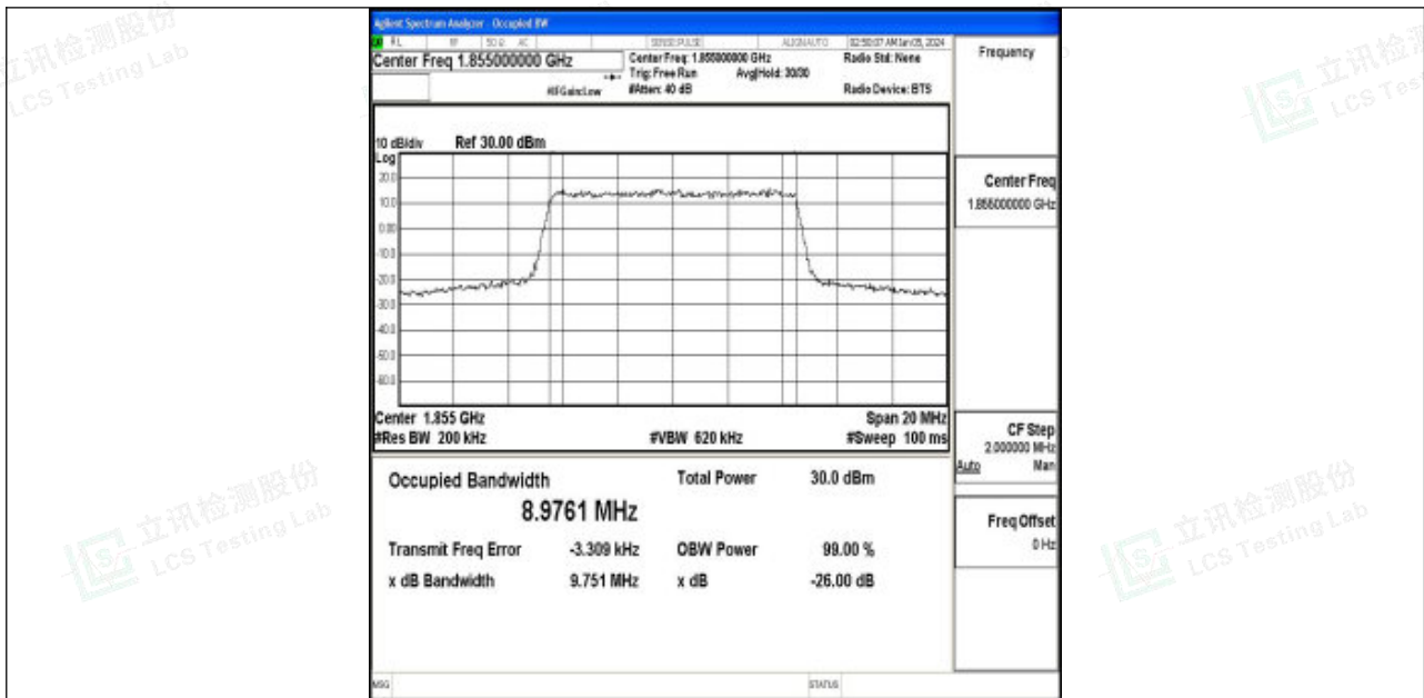
Band2-10MHz-QPSK-18650-50RB#0-PASS
