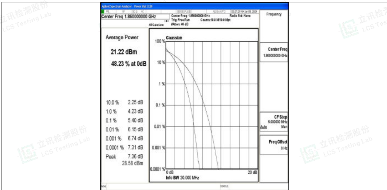
Band2-20MHz-QPSK-18700-100RB#0-PASS
