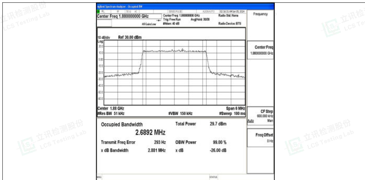
Band2-3MHz-QPSK-18900-15RB#0-PASS
