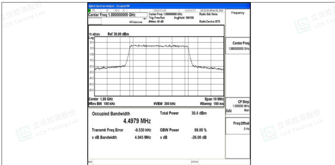
Band2-5MHz-QPSK-18900-25RB#0-PASS
