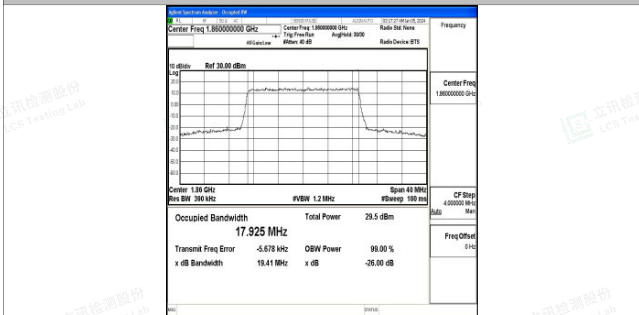
Band2-20MHz-16QAM-18700-100RB#0-PASS
