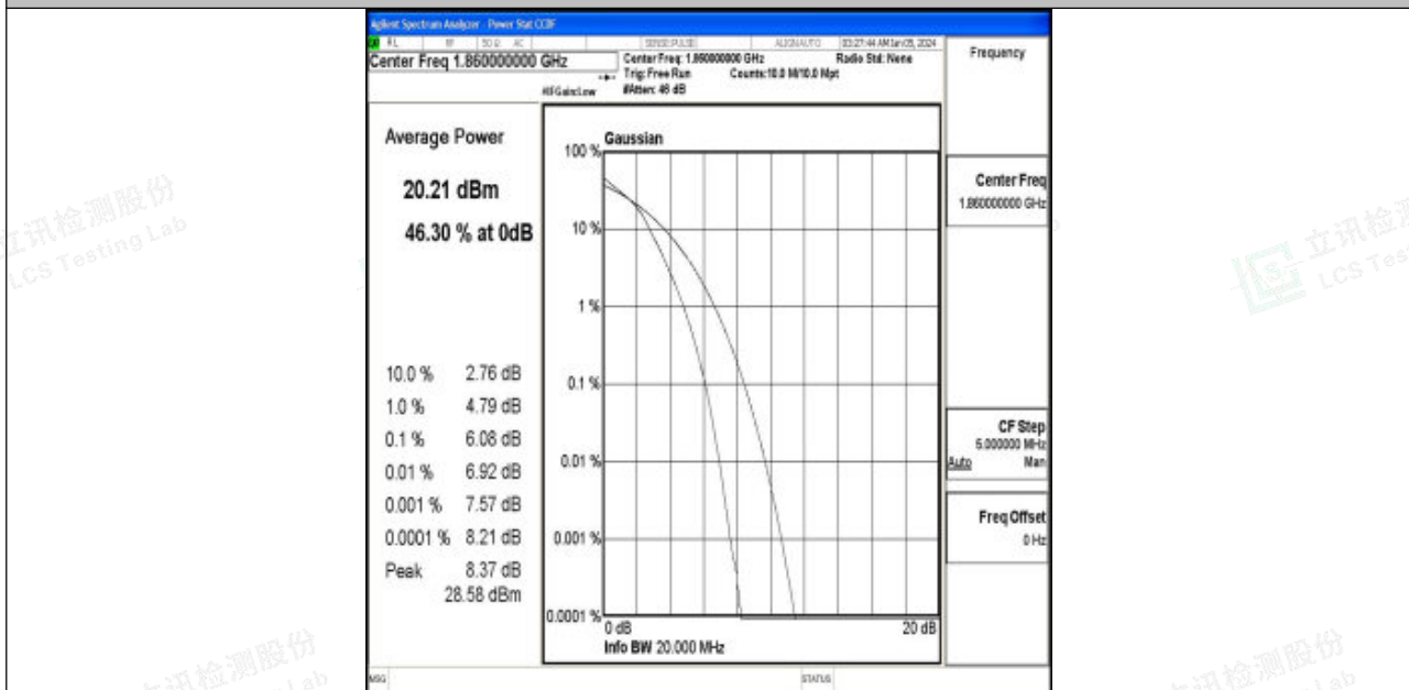
Band2-20MHz-16QAM-18700-100RB#0-PASS
