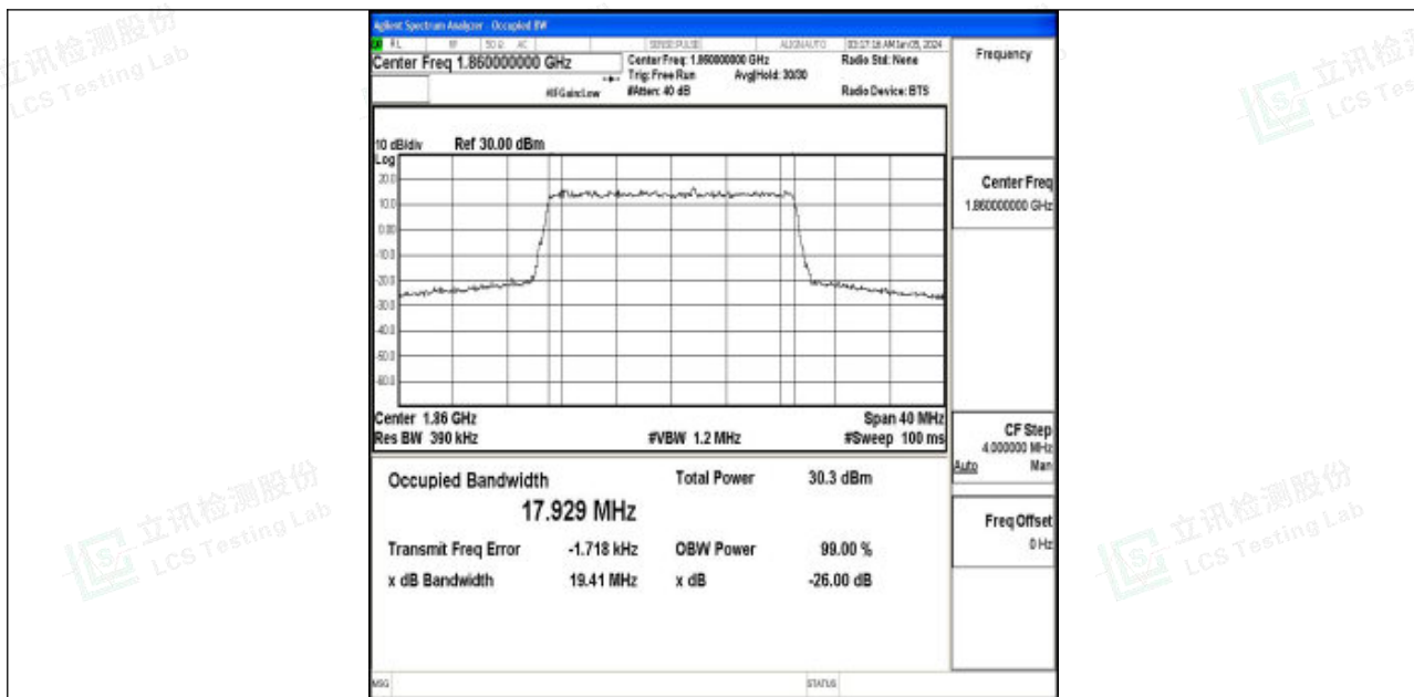
Band2-20MHz-QPSK-18700-100RB#0-PASS
