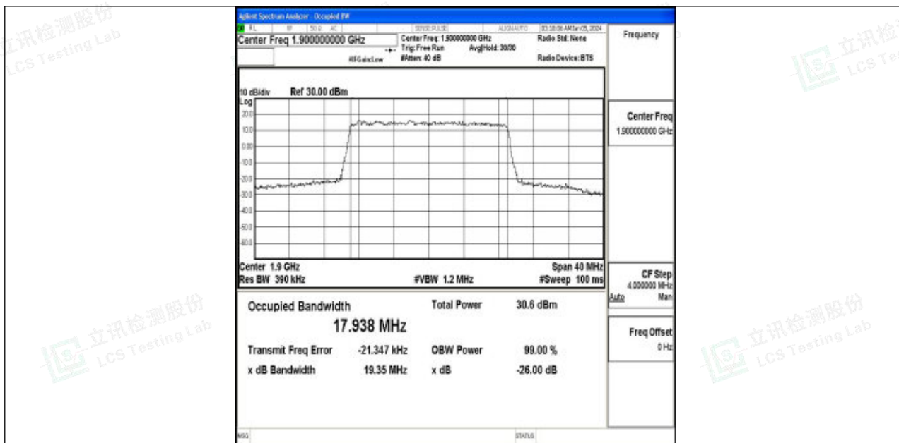
Band2-20MHz-QPSK-19100-100RB#0-PASS
