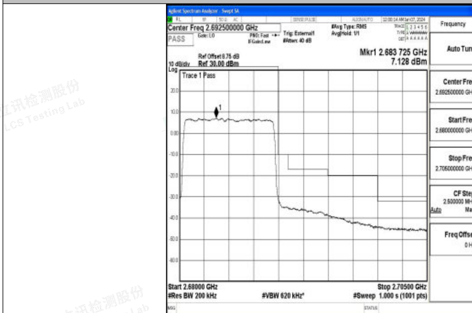
Band41_10MHz_QPSK_41540_50RB#0
