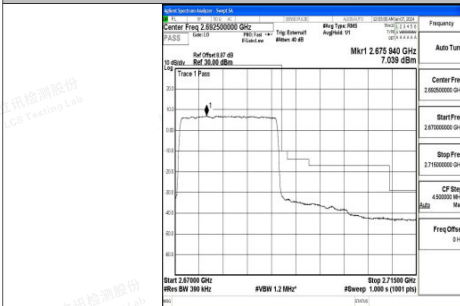
Band41_20MHz_QPSK_41490_100RB#0
