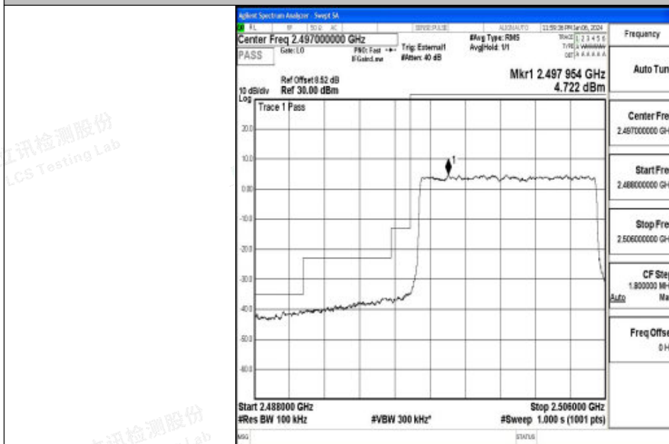
Band41_10MHz_QPSK_39700_50RB#0
