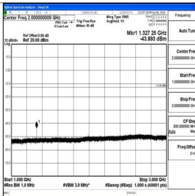
Band71_10MHz_QPSK_133172_1RB#0_1000~3000_1000~3000
