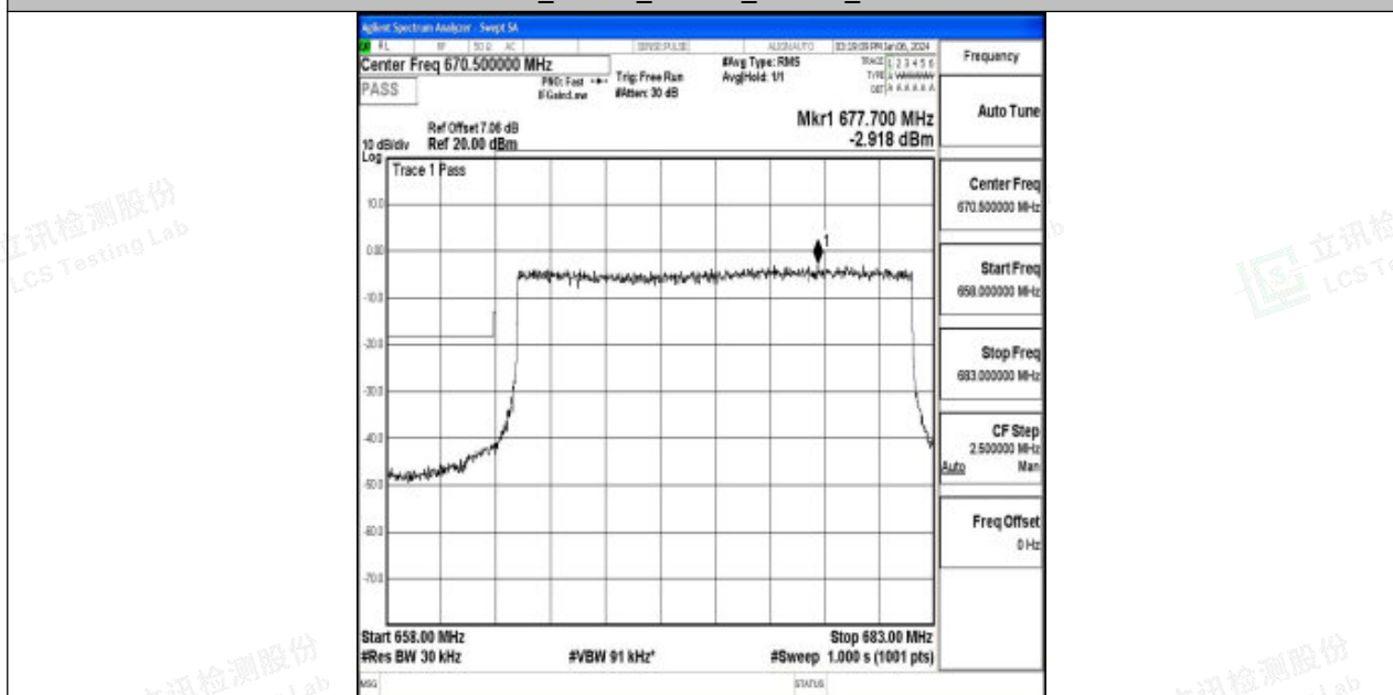
Band71_20MHz_QPSK_133222_100RB#0
