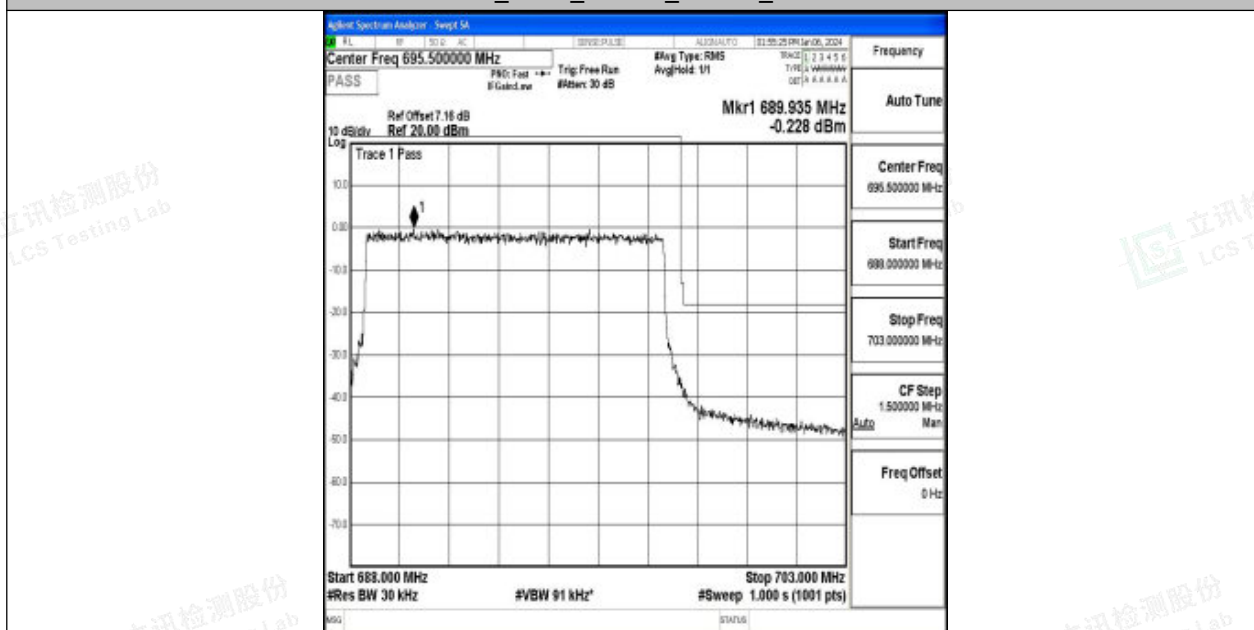
Band71_10MHz_QPSK_133422_50RB#0
