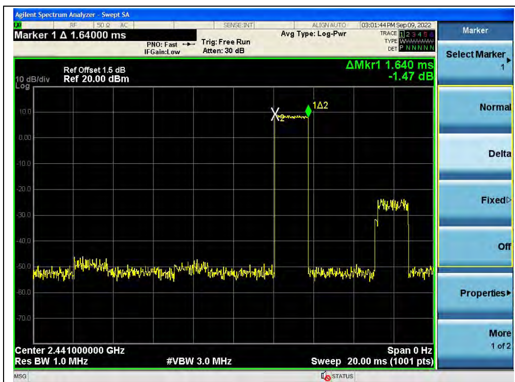
(DH3, 8-DPSK)
