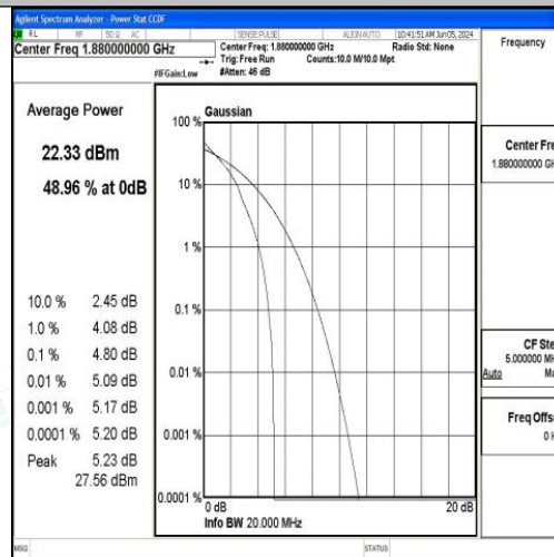
Band2-20MHz-QPSK-18900-1RB#0-PASS
