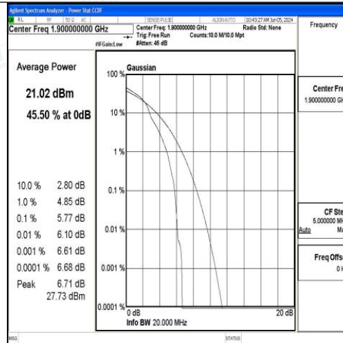
Band2-20MHz-16QAM-19100-1RB#0-PASS
