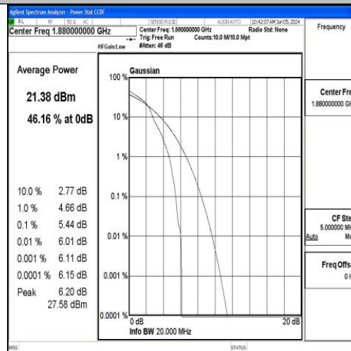
Band2-20MHz-16QAM-18900-1RB#0-PASS
