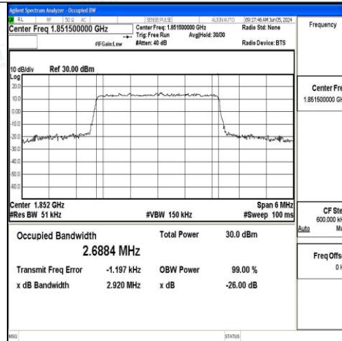
Band2-3MHz-QPSK-18615-15RB#0-PASS
