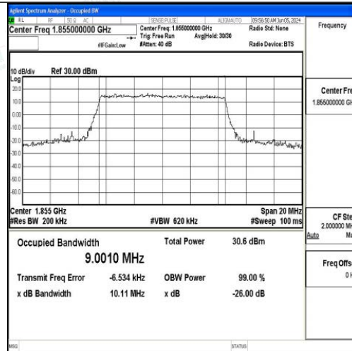
Band2-10MHz-QPSK-18650-50RB#0-PASS
