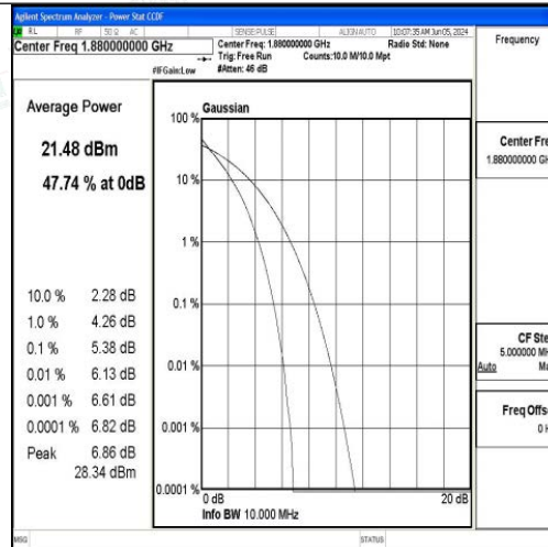
Band2-10MHz-QPSK-18900-50RB#0-PASS
