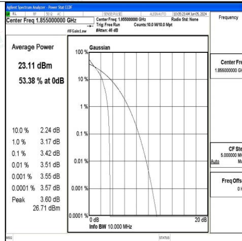
Band2-10MHz-QPSK-18650-1RB#0-PASS
