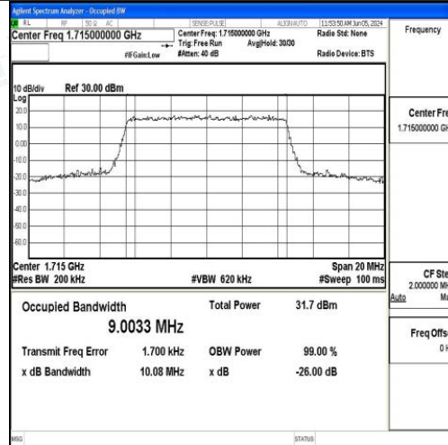
Band4-10MHz-QPSK-20000-50RB#0-PASS
