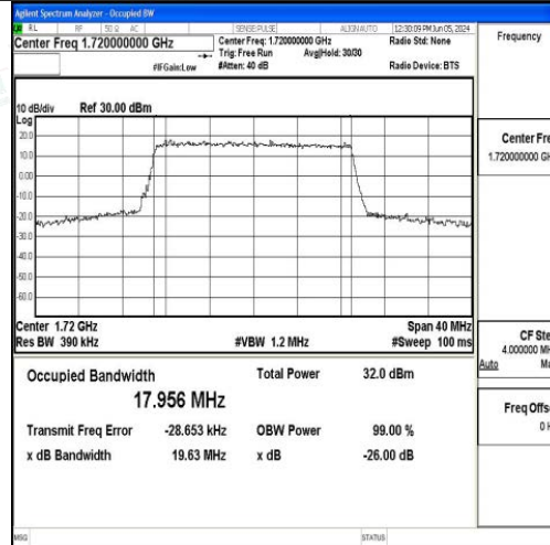
Band4-20MHz-QPSK-20050-100RB#0-PASS
