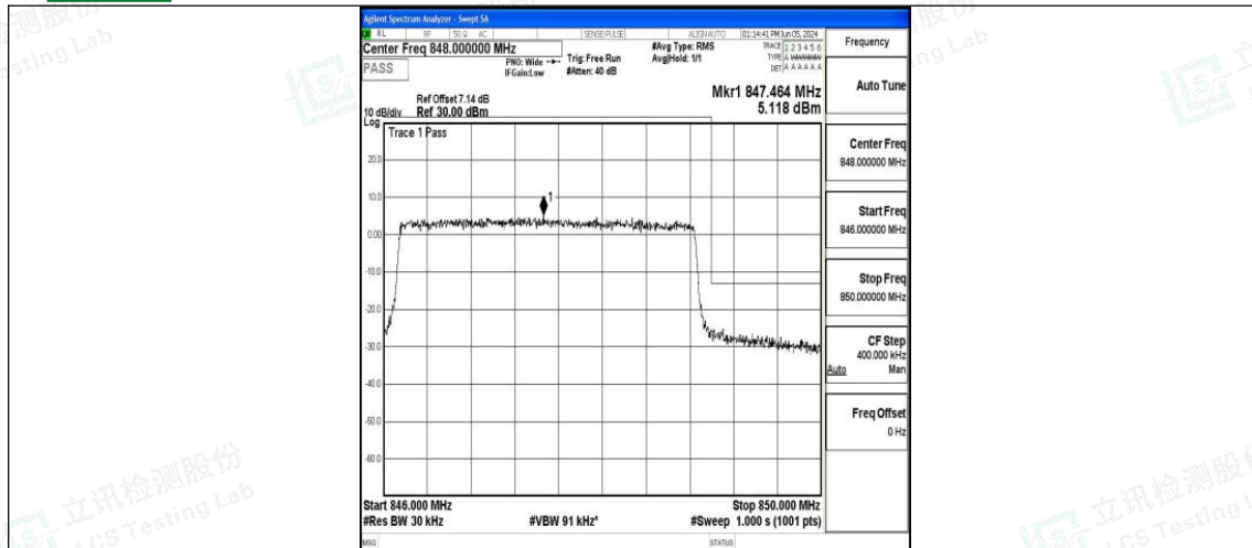
Band5_3MHz_16QAM_20635_15RB#0
