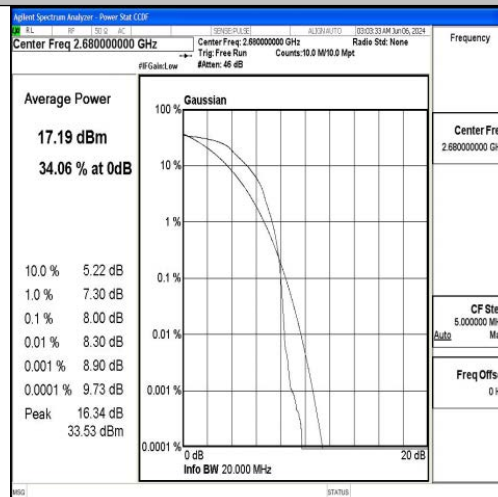
Band41-20MHz-QPSK-41490-1RB#0-PASS
