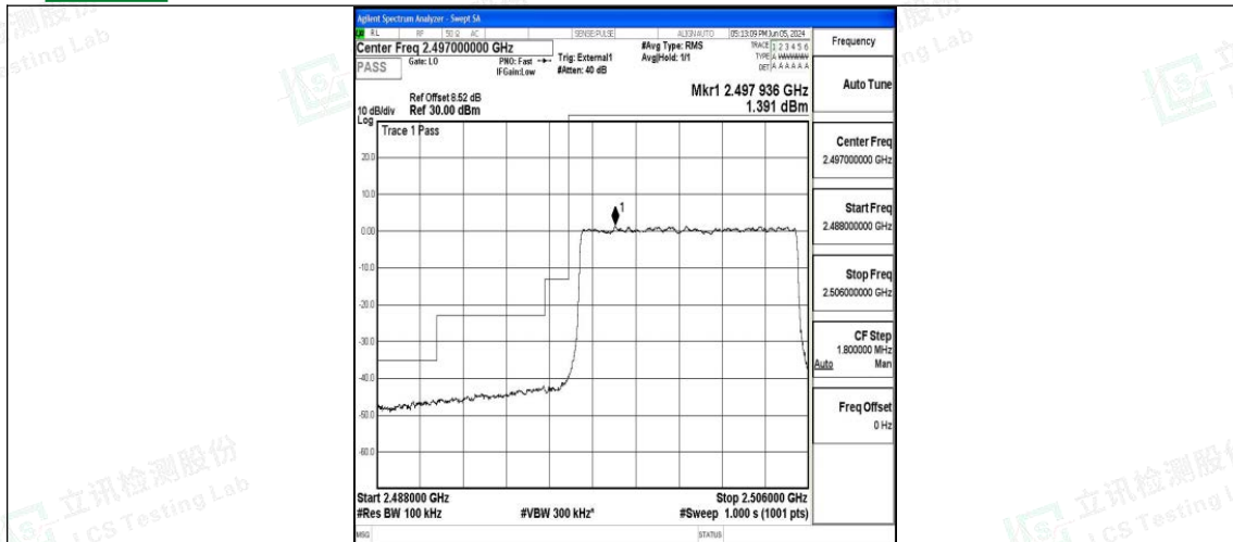
Band41_10MHz_QPSK_39700_50RB#0
