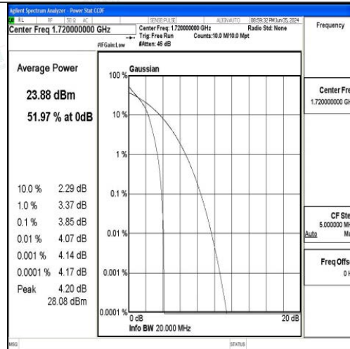
Band66-20MHz-QPSK-132072-1RB#0-PASS
