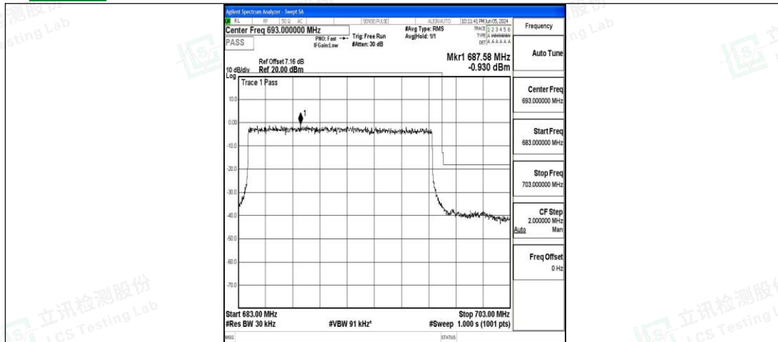
Band71_15MHz_QPSK_133397_75RB#0
