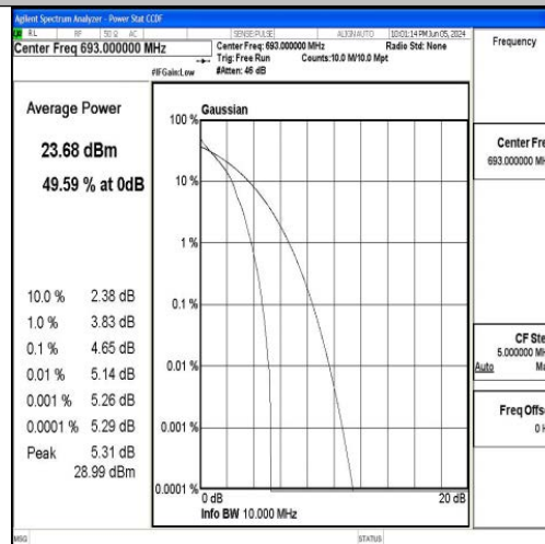
Band71-10MHz-QPSK-133422-1RB#0-PASS
