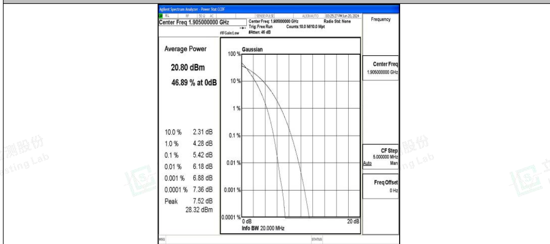
Band25-20MHz-QPSK-26590-100RB#0-PASS
