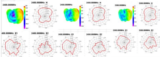
2400.00MHz - 2500.00MHz Gain
