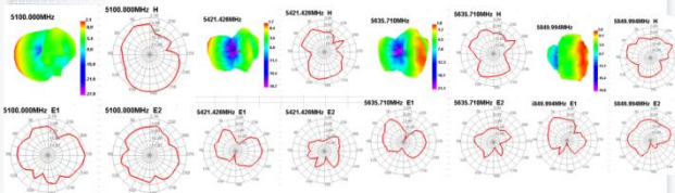
5100.00MHz - 5850.00MHz Gain
