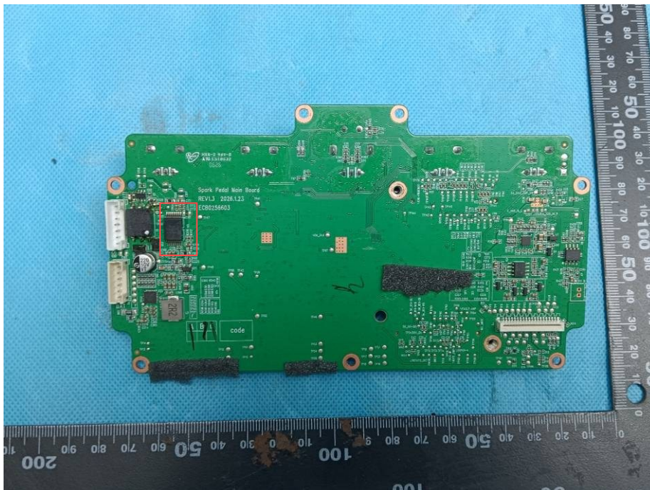
USB port isolator IC option 1: ISOUSB111
