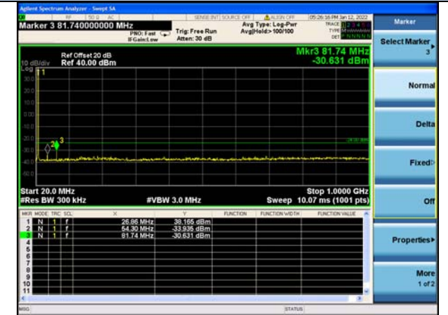
20MHz-1GHz
