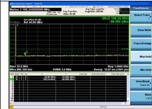
20MHz-1GHz
