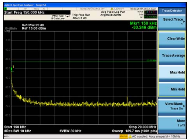
150KHz-20MHz
