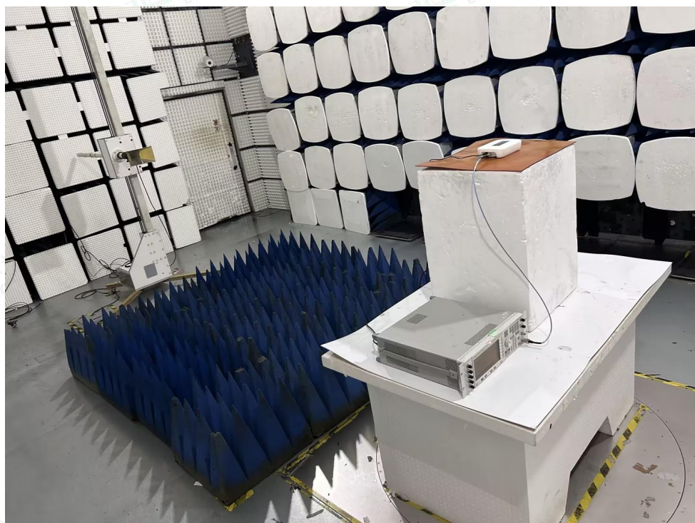
Fig. 2 (Above 1GHz)
