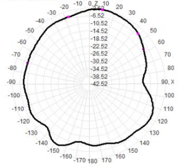
2400.0MHz Total(E1-XZ), Max= -2.65dBi
