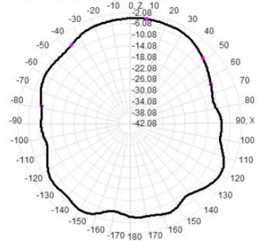
2450.0MHz Total(E1-XZ), Max= -3.97dBi
