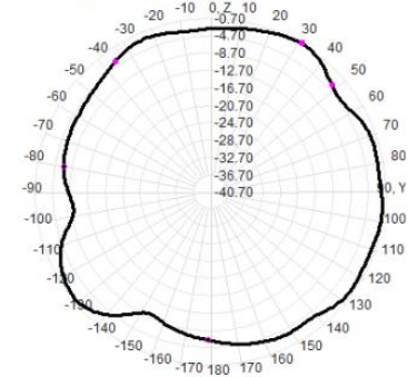
2500.0MHz Total(E2-YZ), Max= -0.70dBi
