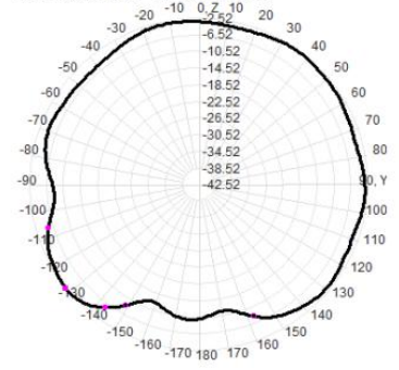
2400.0MHz Total(E2-YZ), Max= -2.52dBi
