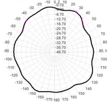
2500.0MHz Total(E1-XZ), Max= -2.18dBi
