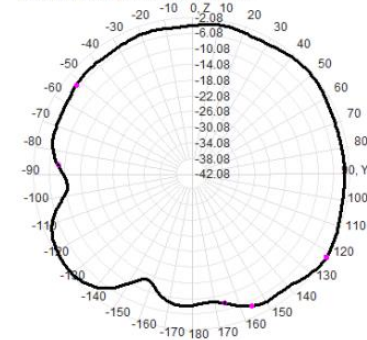
2450.0MHz Total(E2-YZ), Max= -2.08dBi
