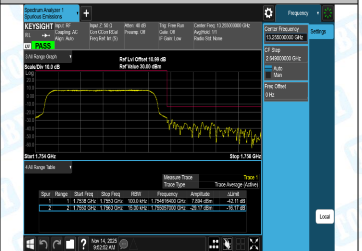
Band4-3MHz-QPSK-19965-1RB#14-PASS
