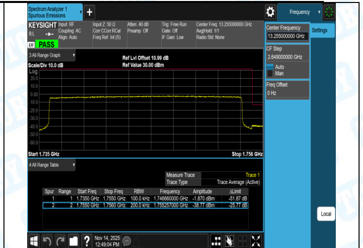
Band4-20MHz-16QAM-20050-1RB#99-PASS
