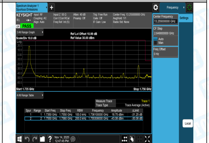
Band4-20MHz-QPSK-20300-1RB#99-PASS
