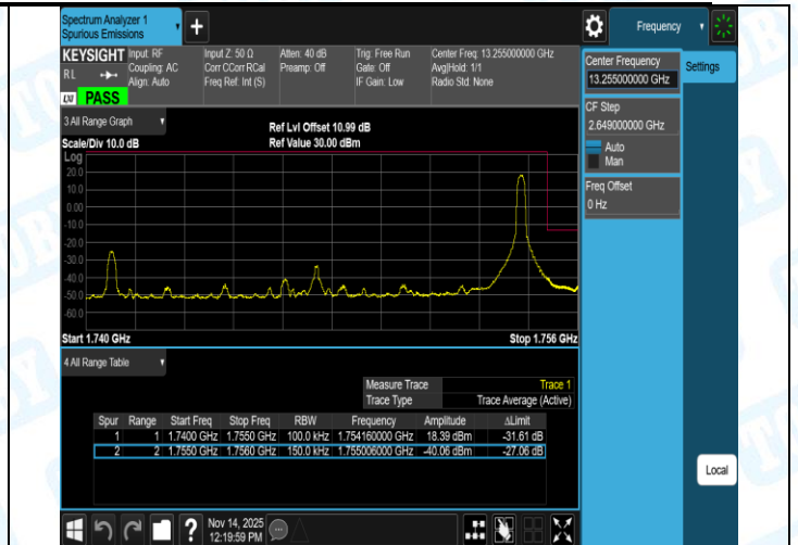
Band4-20MHz-QPSK-20050-1RB#99-PASS
