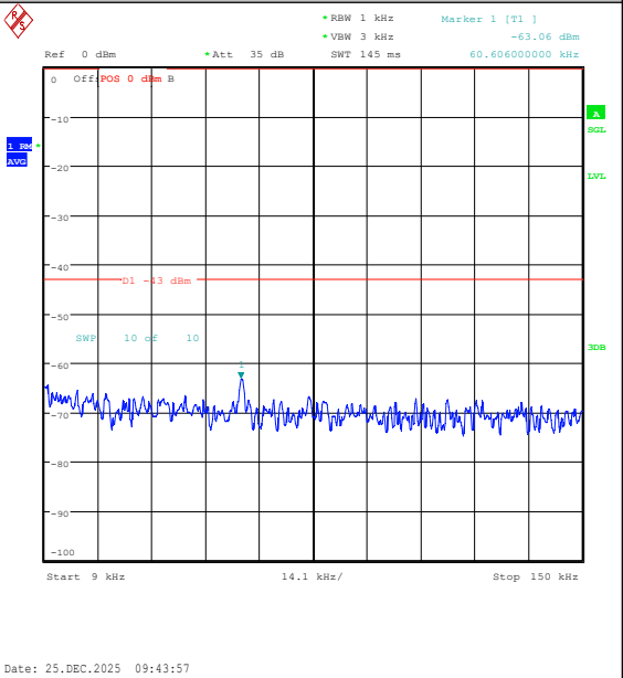
Band4-20MHz-QPSK-20300-100RB#0-0.009~0.15 -PASS
