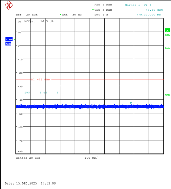
Band41(2535-2655)-5MHz-QPSK-41215-1RB#0-20000~27000-PASS
