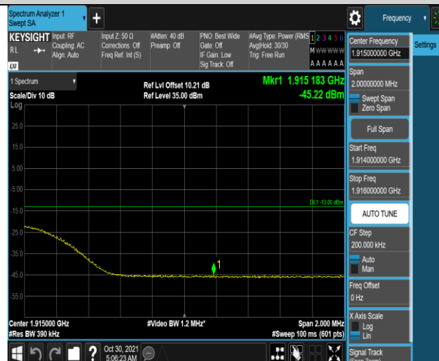
Band25-20MHz-16QAM-26590-1RB#99
