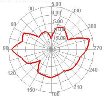
5750.000MHz E1
