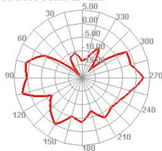
5750.000MHz E2
