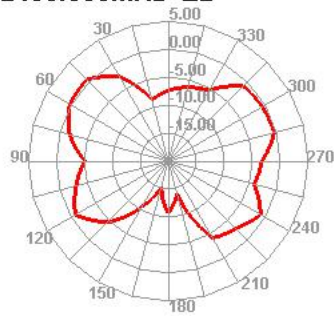
2450.000MHz E2
