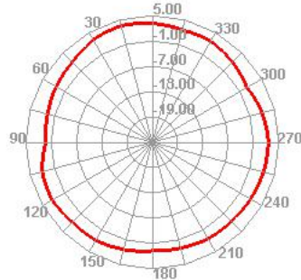
5750.000MHz H
