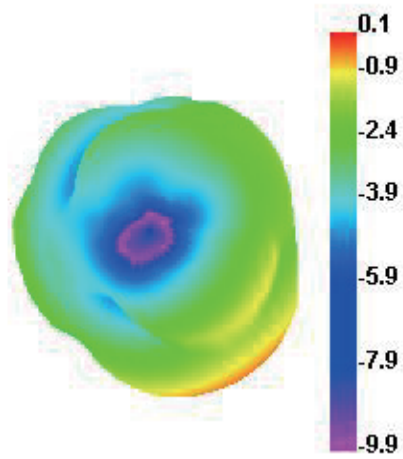
2450.000MHz
