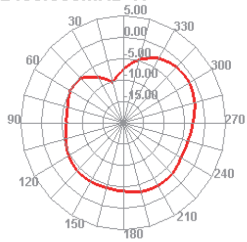
2450.000MHz H
