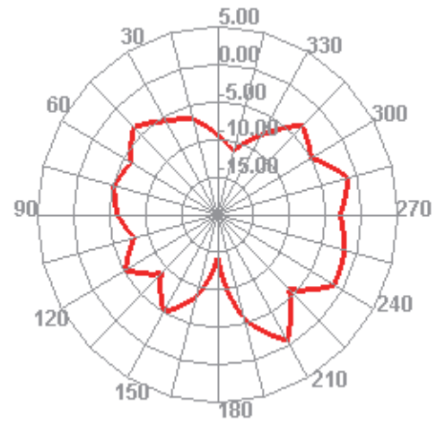
2450.000MHz E2
