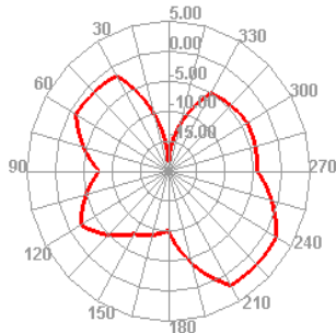
2400.000MHz E1
