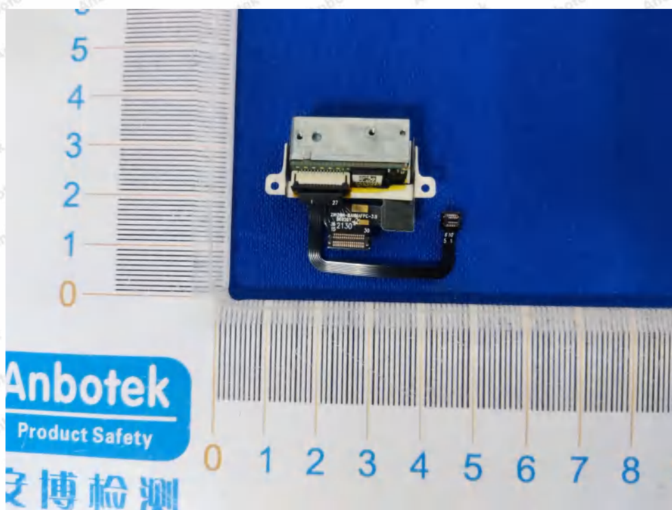
NFC ANT
