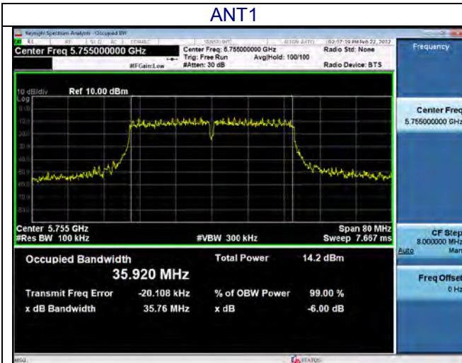
CH151 -5755MHz
