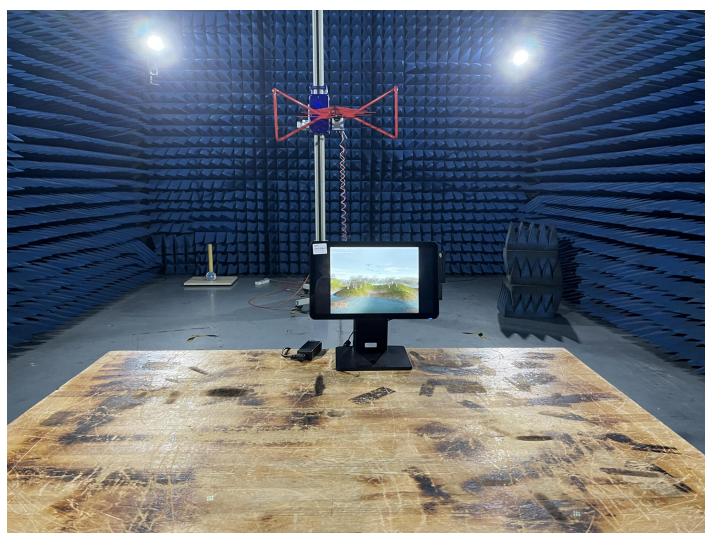
(30M-1G)
