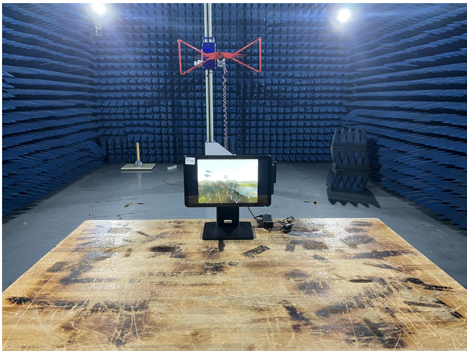
(30M-1G)
