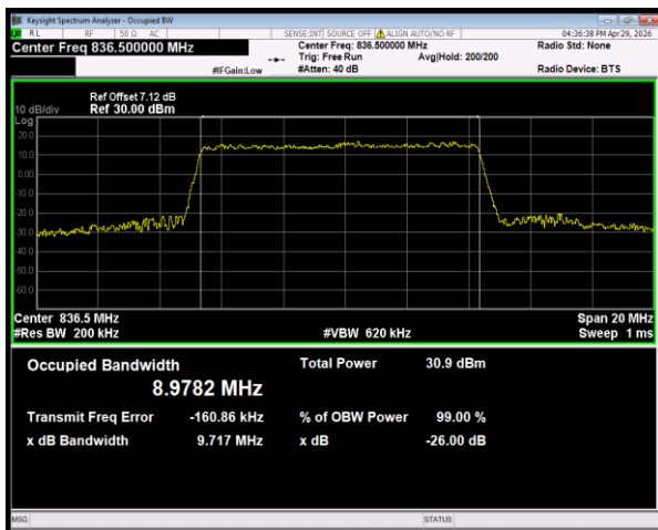
n5 SCS=15kHz DFT_QPSK BW=10MHz Channel=167300 RB=50@0
