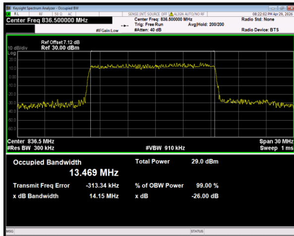
n26(824-849) SCS=15kHz DFT_QPSK BW=15MHz Channel=167300 RB=75@0
