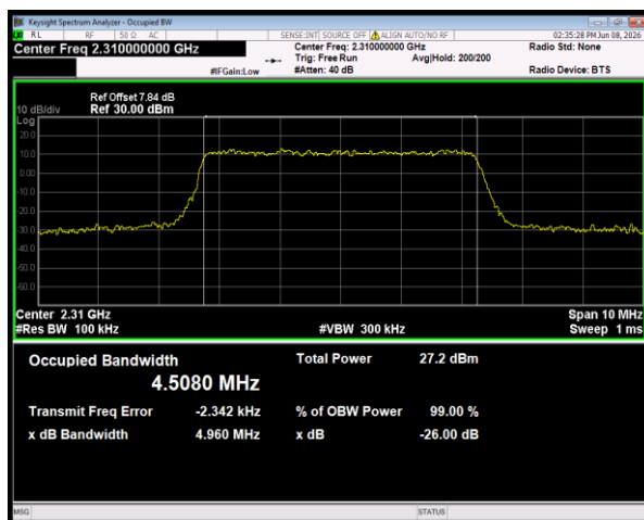
n30 SCS=15kHz CP_16QAM BW=5MHz Channel=462000 RB=25@0
