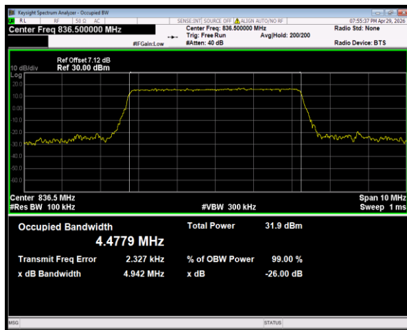
n26(824-849) SCS=15kHz DFT_QPSK BW=5MHz Channel=167300 RB=25@0
