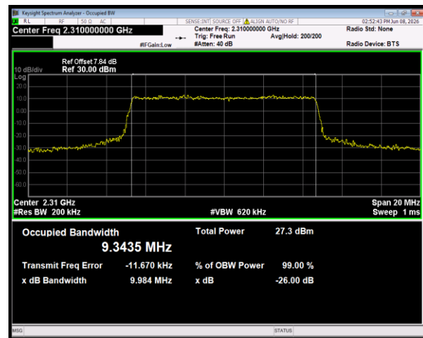
n30 SCS=15kHz CP_16QAM BW=10MHz Channel=462000 RB=52@0
