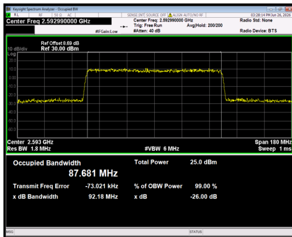
n41 SCS=30kHz CP_16QAM BW=90MHz Channel=518598 RB=245@0
