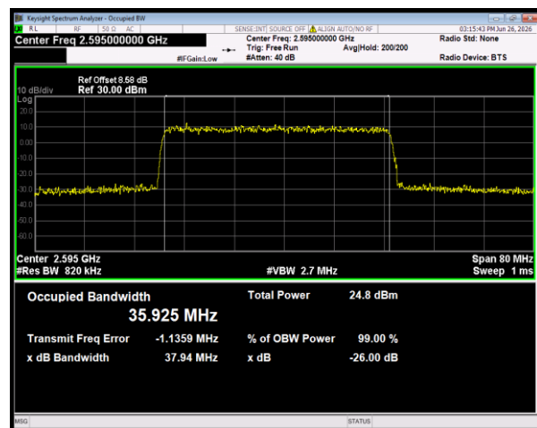
n38 SCS=30kHz DFT_QPSK BW=40MHz Channel=519000 RB=100@0
