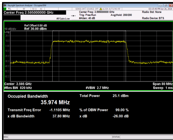
n38 SCS=30kHz DFT_BPSK BW=40MHz Channel=519000 RB=100@0
