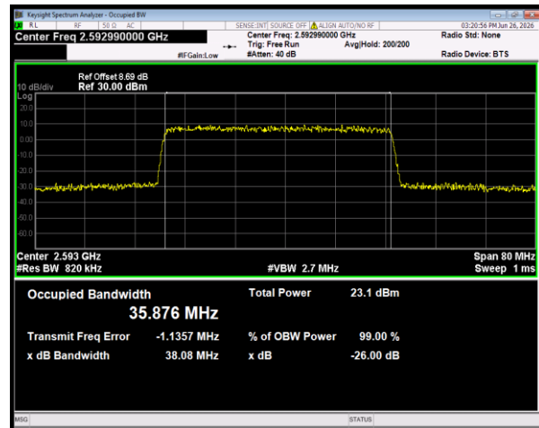
n41 SCS=30kHz DFT_256QAM BW=40MHz Channel=518598 RB=100@0
