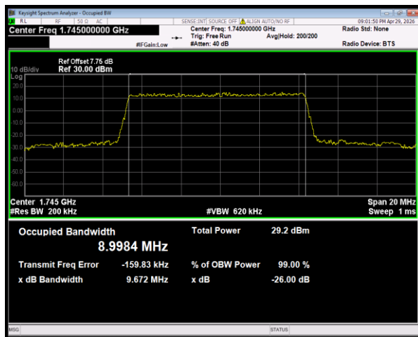
n66 SCS=15kHz DFT_QPSK BW=10MHz Channel=349000 RB=50@0
