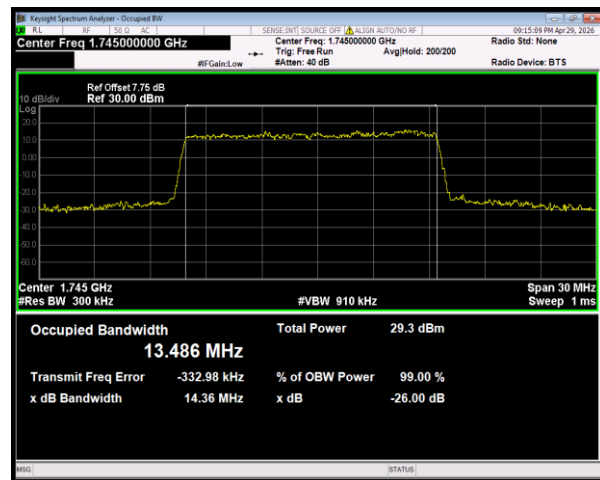
n66 SCS=15kHz DFT_QPSK BW=15MHz Channel=349000 RB=75@0
