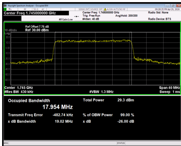
n66 SCS=15kHz DFT_QPSK BW=20MHz Channel=349000 RB=100@0
