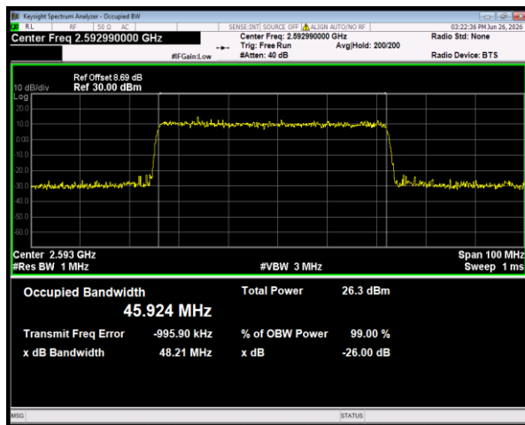
n41 SCS=30kHz DFT_QPSK BW=50MHz Channel=518598 RB=128@0
