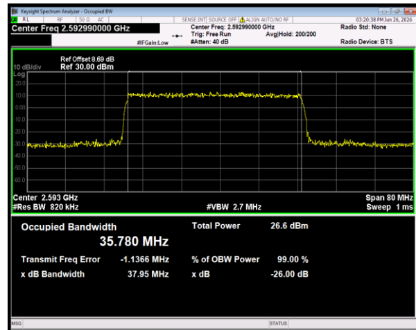
n41 SCS=30kHz DFT_QPSK BW=40MHz Channel=518598 RB=100@0
