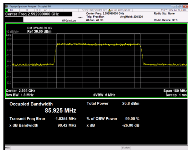
n41 SCS=30kHz DFT_QPSK BW=90MHz Channel=518598 RB=240@0
