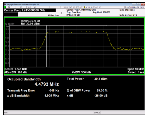
n66 SCS=15kHz DFT_QPSK BW=5MHz Channel=349000 RB=25@0
