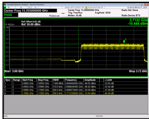
n78(3700-3800) SCS=30kHz DFT_16QAM BW=20MHz LowChannel=647334 RB=50@0
