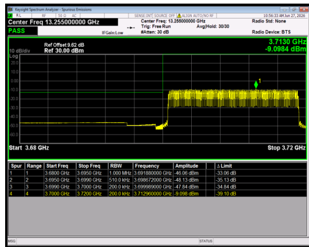
n78(3700-3800) SCS=30kHz DFT_BPSK BW=20MHz LowChannel=647334 RB=50@0
