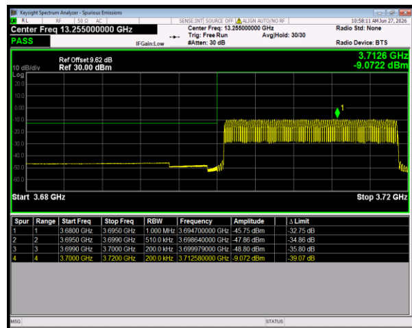
n78(3700-3800) SCS=30kHz DFT_QPSK BW=20MHz LowChannel=647334 RB=50@0
