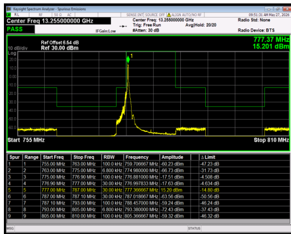
n13 SCS=15kHz DFT_16QAM BW=10MHz LowChannel=156400 RB=1@0
