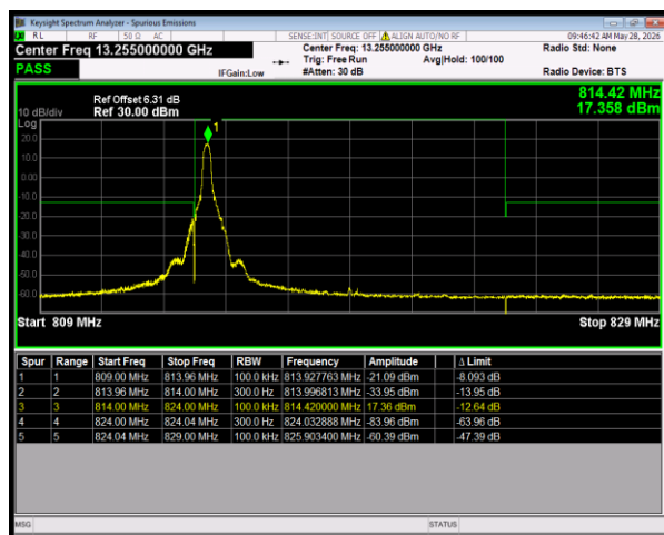
n26(814-824) SCS=15kHz CP_QPSK BW=10MHz LowChannel=163800 RB=1@0
