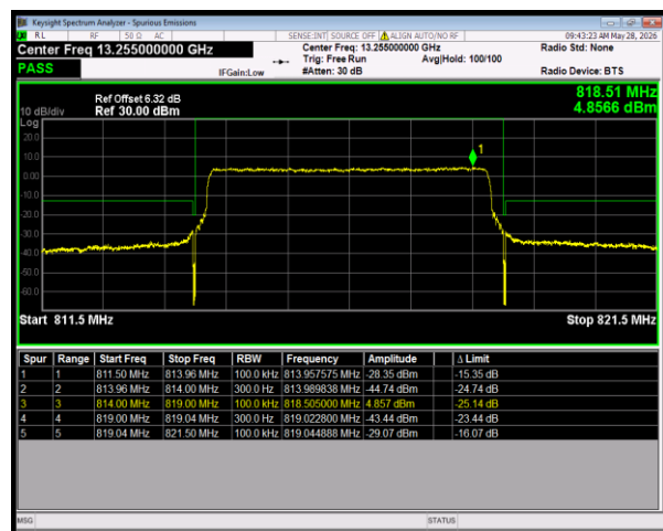
n26(814-824) SCS=15kHz CP_16QAM BW=5MHz LowChannel=163300 RB=25@0
