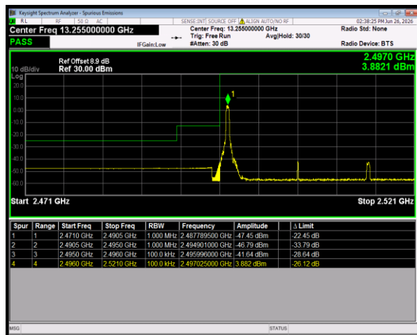
n41 SCS=30kHz CP_QPSK BW=20MHz LowChannel=501204 RB=1@0
