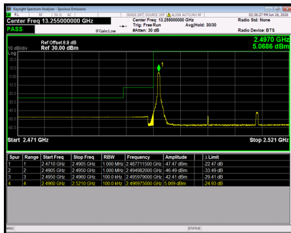
n41 SCS=30kHz DFT_QPSK BW=20MHz LowChannel=501204 RB=1@0
