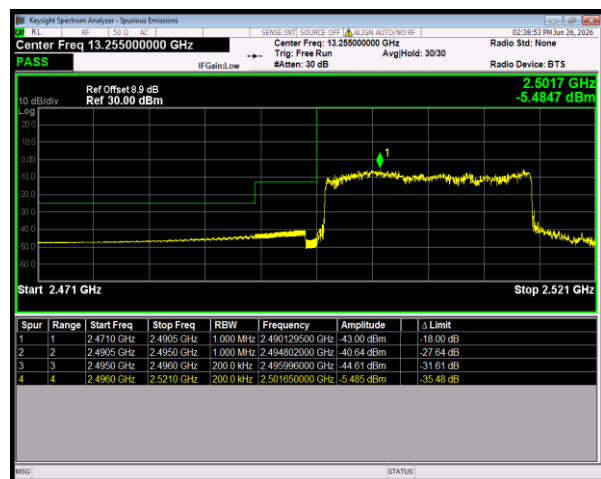
n41 SCS=30kHz CP_16QAM BW=20MHz LowChannel=501204 RB=51@0
