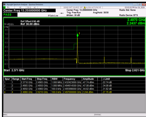
n41 SCS=30kHz CP_16QAM BW=100MHz LowChannel=509202 RB=1@0
