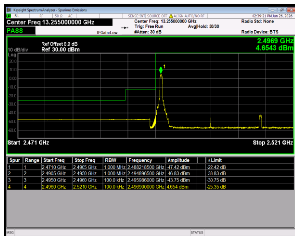
n41 SCS=30kHz CP_16QAM BW=20MHz LowChannel=501204 RB=1@0
