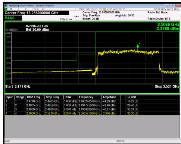
n41 SCS=30kHz DFT_QPSK BW=20MHz LowChannel=501204 RB=50@0
