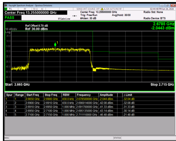
n41 SCS=30kHz CP_16QAM BW=20MHz HighChannel=535998 RB=51@0
