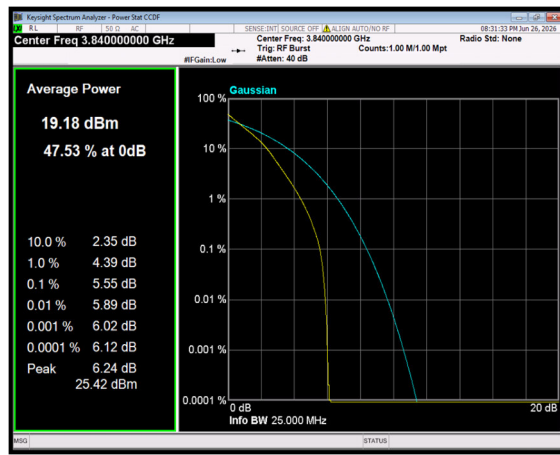
n77(3700-3980) SCS=30kHz DFT_QPSK BW=20MHz Channel=656000 RB=50@0
