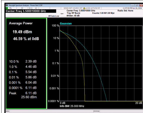
n77(3450-3550) SCS=30kHz DFT_QPSK BW=20MHz Channel=633334 RB=50@0
