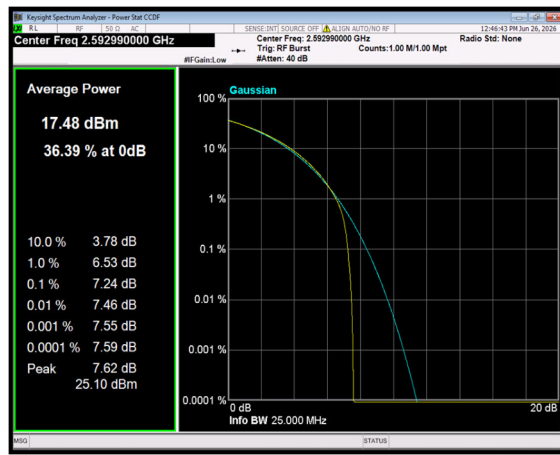
n41 SCS=30kHz CP_16QAM BW=20MHz Channel=518598 RB=51@0
