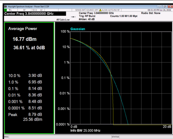
n77(3700-3980) SCS=30kHz CP_16QAM BW=20MHz Channel=656000 RB=51@0
