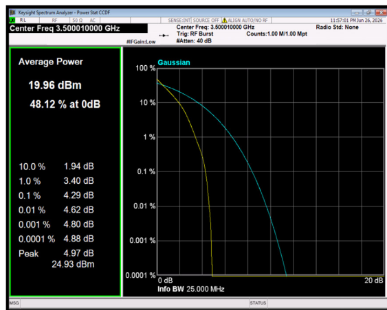
n77(3450-3550) SCS=30kHz DFT_BPSK BW=20MHz Channel=633334 RB=50@0
