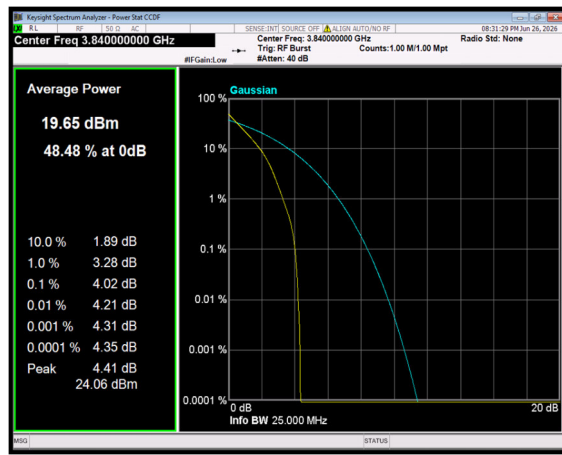
n77(3700-3980) SCS=30kHz DFT_BPSK BW=20MHz Channel=656000 RB=50@0
