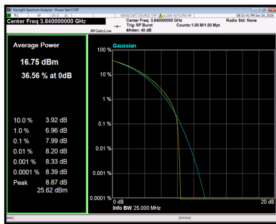
n77(3700-3980) SCS=30kHz CP_QPSK BW=20MHz Channel=656000 RB=51@0
