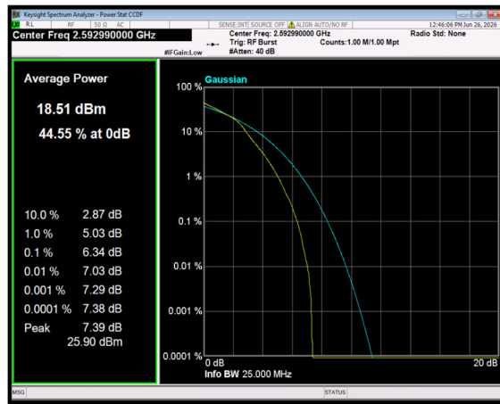
n41 SCS=30kHz DFT_16QAM BW=20MHz Channel=518598 RB=50@0
