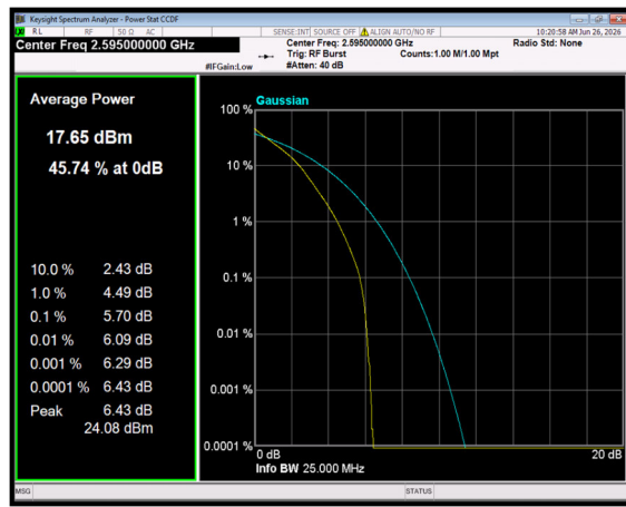
n38 SCS=30kHz DFT_QPSK BW=20MHz Channel=519000 RB=50@0
