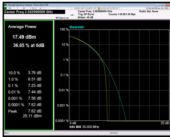
n41 SCS=30kHz CP_QPSK BW=20MHz Channel=518598 RB=51@0
