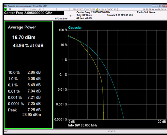
n38 SCS=30kHz DFT_16QAM BW=20MHz Channel=519000 RB=50@0
