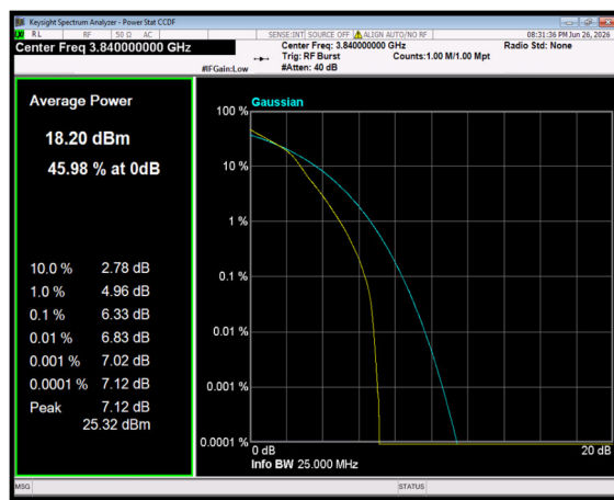
n77(3700-3980) SCS=30kHz DFT_16QAM BW=20MHz Channel=656000 RB=50@0
