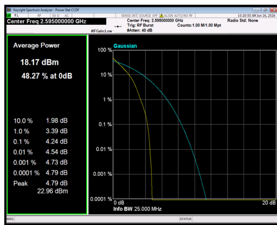
n38 SCS=30kHz DFT_BPSK BW=20MHz Channel=519000 RB=50@0
