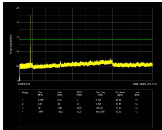
n5 SCS=15kHz CP_QPSK BW=5MHz Channel=165300 RB=25@0
