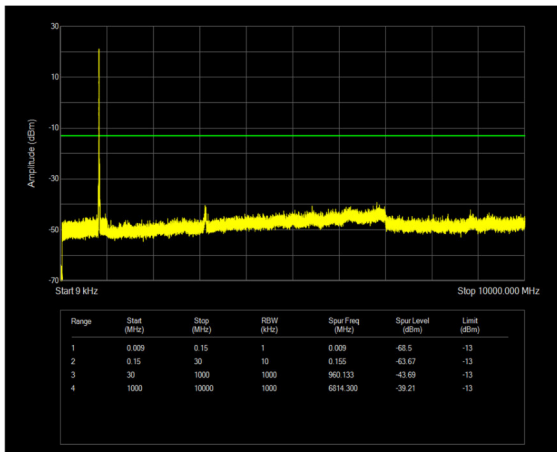
n5 SCS=15kHz DFT_QPSK BW=5MHz Channel=165300 RB=25@0
