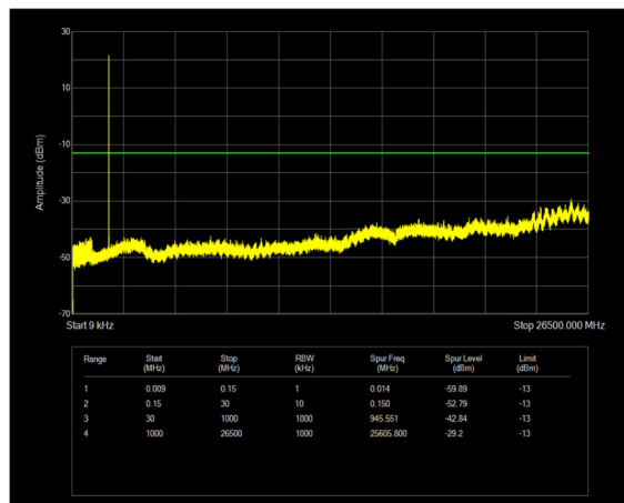
n2 SCS=15kHz DFT_QPSK BW=20MHz Channel=376000 RB=1@0
