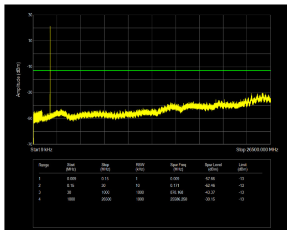
n2 SCS=15kHz CP_QPSK BW=10MHz Channel=376000 RB=1@51
