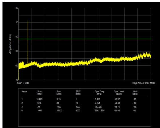
n2 SCS=15kHz CP_QPSK BW=10MHz Channel=371000 RB=52@0
