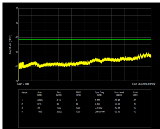
n2 SCS=15kHz CP_QPSK BW=10MHz Channel=376000 RB=52@0
