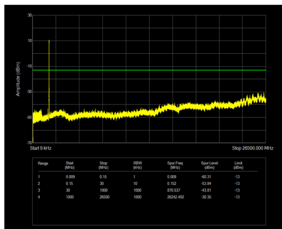
n2 SCS=15kHz DFT_QPSK BW=20MHz Channel=372000 RB=100@0
