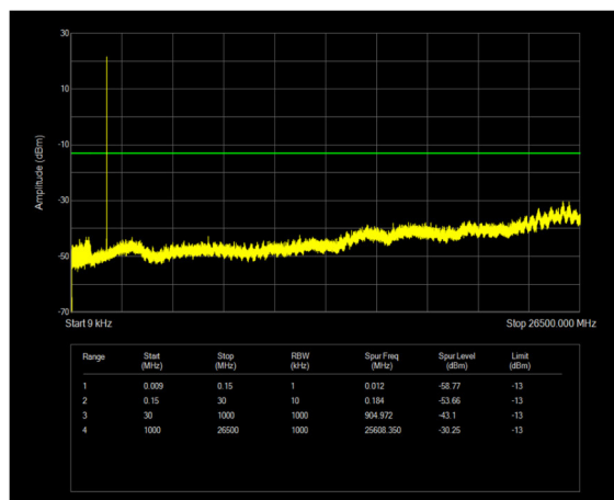
n2 SCS=15kHz DFT_QPSK BW=20MHz Channel=372000 RB=1@0
