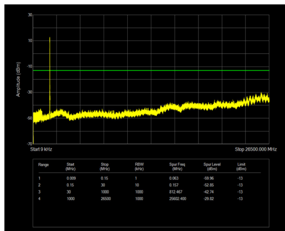
n2 SCS=15kHz DFT_QPSK BW=20MHz Channel=376000 RB=100@0
