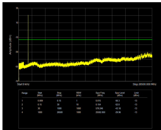
n2 SCS=15kHz CP_QPSK BW=10MHz Channel=376000 RB=1@0
