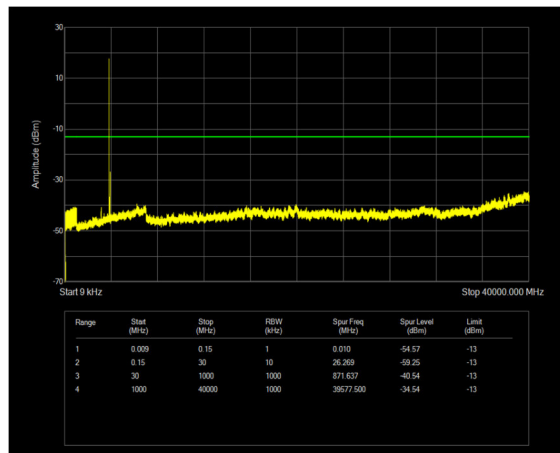
n77(3700-3980) SCS=30kHz CP_QPSK BW=100MHz Channel=656000 RB=1@0
