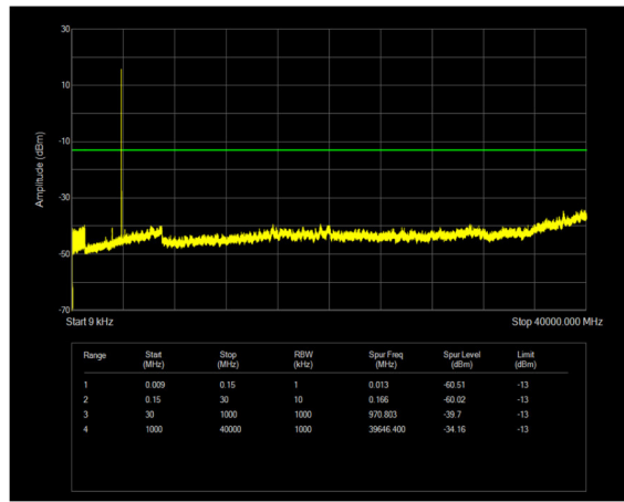
n77(3700-3980) SCS=30kHz CP_QPSK BW=20MHz Channel=656000 RB=1@0
