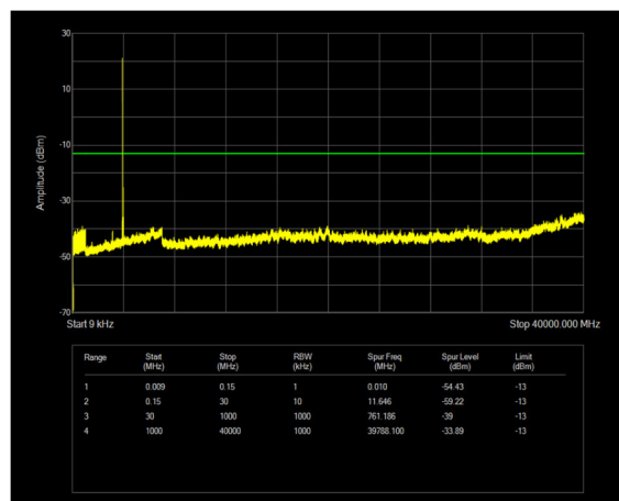
n77(3700-3980) SCS=30kHz CP_QPSK BW=100MHz Channel=662000 RB=1@0
