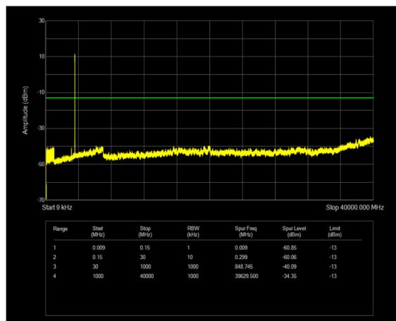
n77(3450-3550) SCS=30kHz DFT_QPSK BW=20MHz Channel=636000 RB=50@0
