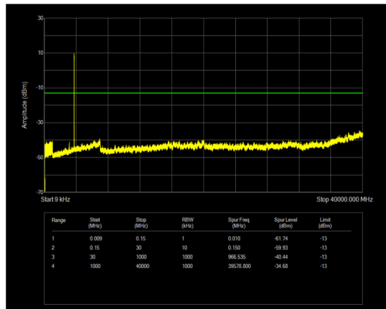
n77(3700-3980) SCS=30kHz CP_QPSK BW=20MHz Channel=647334 RB=51@0
