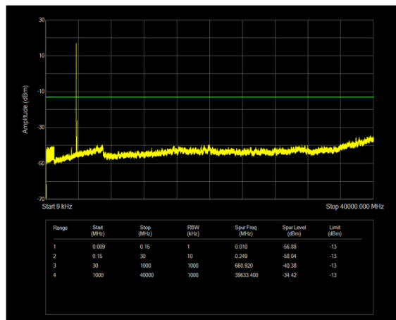
n77(3700-3980) SCS=30kHz CP_QPSK BW=100MHz Channel=650000 RB=1@0
