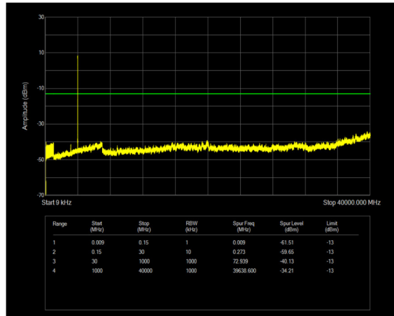
n77(3700-3980) SCS=30kHz CP_QPSK BW=20MHz Channel=664666 RB=51@0
