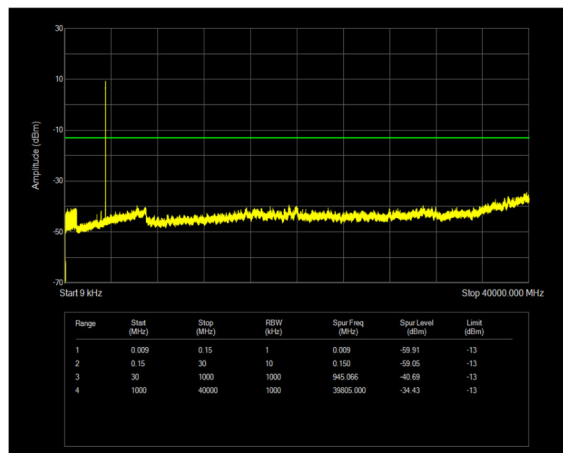
n77(3450-3550) SCS=30kHz DFT_QPSK BW=20MHz Channel=633334 RB=50@0
