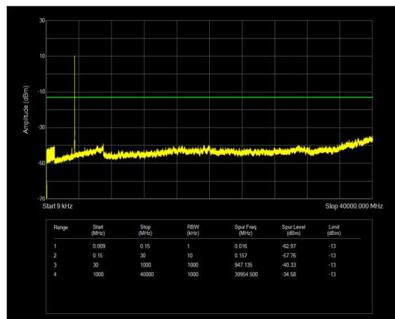
n77(3450-3550) SCS=30kHz DFT_QPSK BW=20MHz Channel=630668 RB=50@0
