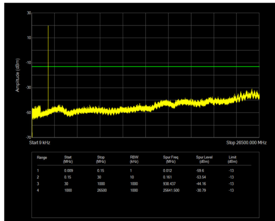
n25 SCS=15kHz CP_QPSK BW=20MHz Channel=381000 RB=1@0
