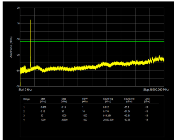
n25 SCS=15kHz DFT_QPSK BW=10MHz Channel=376500 RB=50@0
