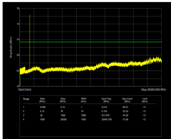
n25 SCS=15kHz DFT_QPSK BW=5MHz Channel=370500 RB=1@0
