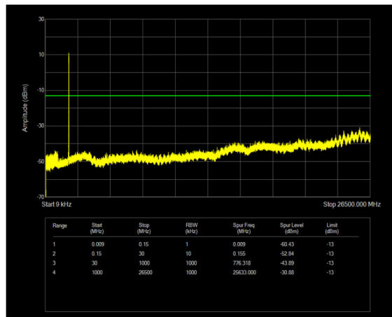
n25 SCS=15kHz CP_QPSK BW=20MHz Channel=381000 RB=106@0
