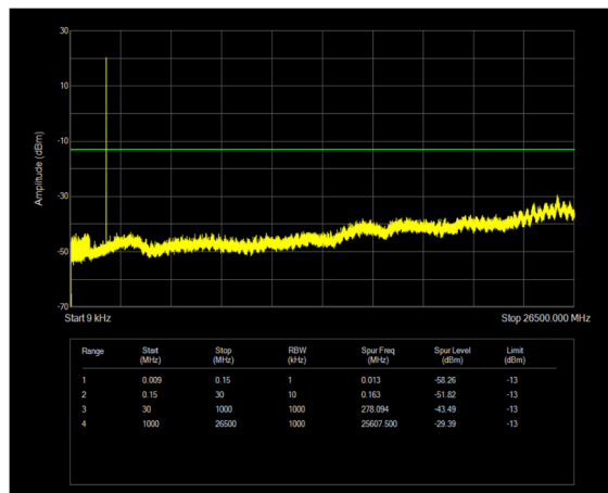
n25 SCS=15kHz CP_QPSK BW=20MHz Channel=376500 RB=1@0
