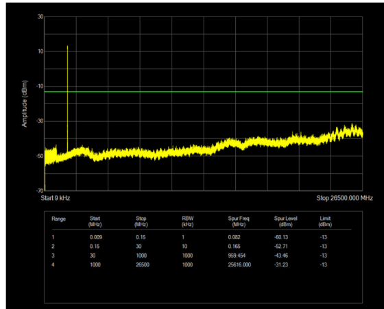
n25 SCS=15kHz DFT_QPSK BW=10MHz Channel=382000 RB=50@0
