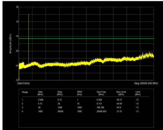
n25 SCS=15kHz DFT_QPSK BW=10MHz Channel=382000 RB=1@51
