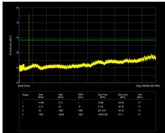
n25 SCS=15kHz CP_QPSK BW=20MHz Channel=381000 RB=1@105
