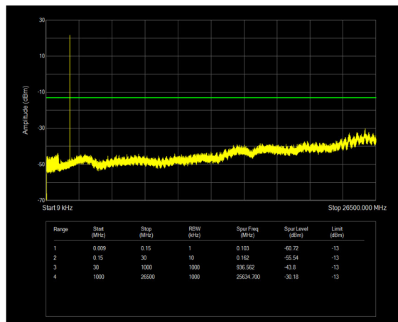
n25 SCS=15kHz DFT_QPSK BW=20MHz Channel=381000 RB=1@0
