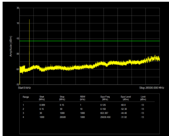
n25 SCS=15kHz DFT_QPSK BW=5MHz Channel=370500 RB=25@0
