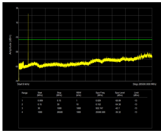
n25 SCS=15kHz DFT_QPSK BW=10MHz Channel=376500 RB=1@51
