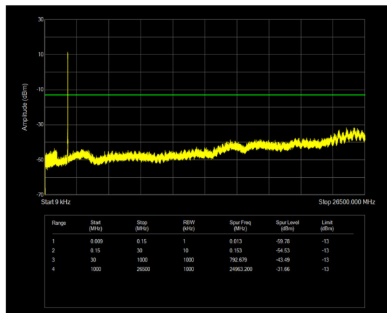
n25 SCS=15kHz DFT_QPSK BW=20MHz Channel=381000 RB=100@0
