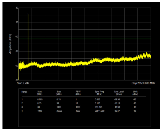
n25 SCS=15kHz DFT_QPSK BW=20MHz Channel=381000 RB=1@105
