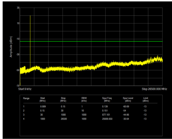
n25 SCS=15kHz DFT_QPSK BW=10MHz Channel=382000 RB=1@0
