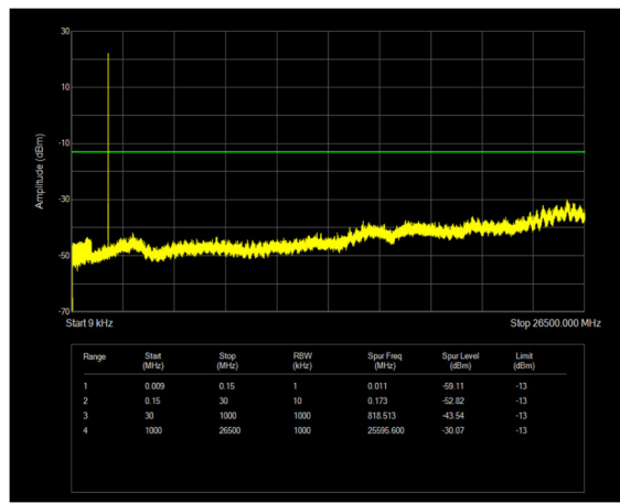
n25 SCS=15kHz DFT_QPSK BW=10MHz Channel=376500 RB=1@0
