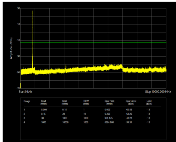
n26(824-849) SCS=15kHz CP_QPSK BW=20MHz Channel=167800 RB=1@105
