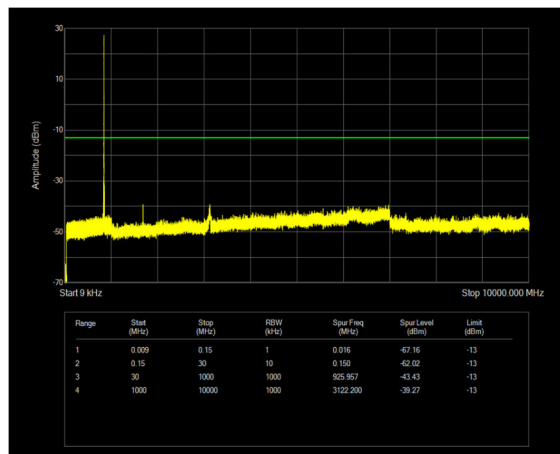
n26(824-849) SCS=15kHz DFT_QPSK BW=10MHz Channel=167300 RB=1@51
