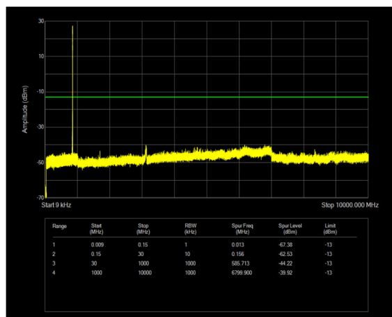
n26(824-849) SCS=15kHz CP_QPSK BW=10MHz Channel=168800 RB=1@51
