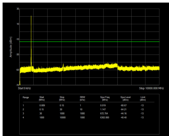
n26(824-849) SCS=15kHz CP_QPSK BW=5MHz Channel=165300 RB=25@0
