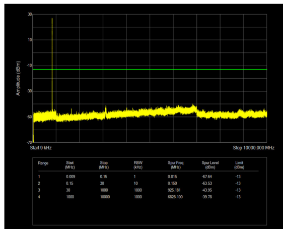
n26(824-849) SCS=15kHz CP_QPSK BW=5MHz Channel=165300 RB=1@0
