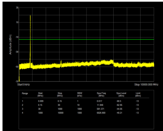
n26(824-849) SCS=15kHz DFT_QPSK BW=10MHz Channel=168800 RB=50@0
