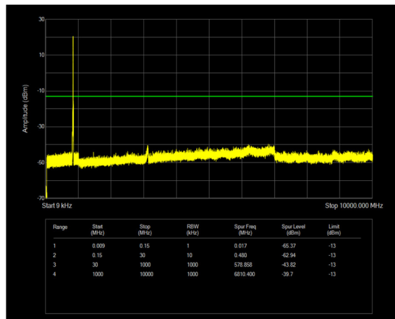
n26(824-849) SCS=15kHz DFT_QPSK BW=10MHz Channel=167300 RB=50@0
