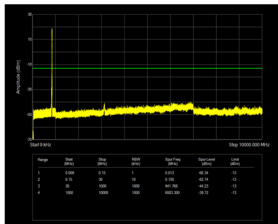
n26(824-849) SCS=15kHz CP_QPSK BW=10MHz Channel=168800 RB=52@0
