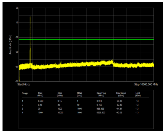
n26(824-849) SCS=15kHz CP_QPSK BW=10MHz Channel=165800 RB=52@0
