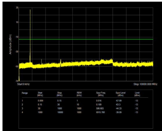
n26(824-849) SCS=15kHz DFT_QPSK BW=20MHz Channel=167300 RB=1@105
