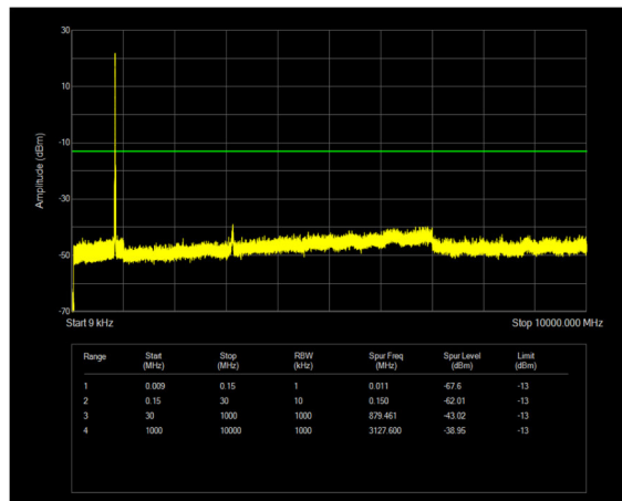
n26(824-849) SCS=15kHz DFT_QPSK BW=5MHz Channel=167300 RB=25@0
