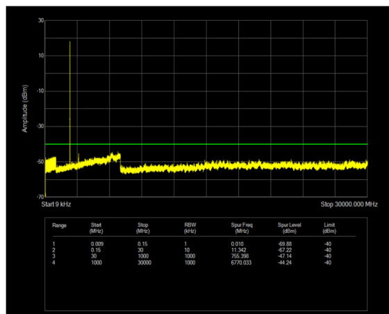
n30 SCS=15kHz CP_QPSK BW=5MHz Channel=461500 RB=25@0
