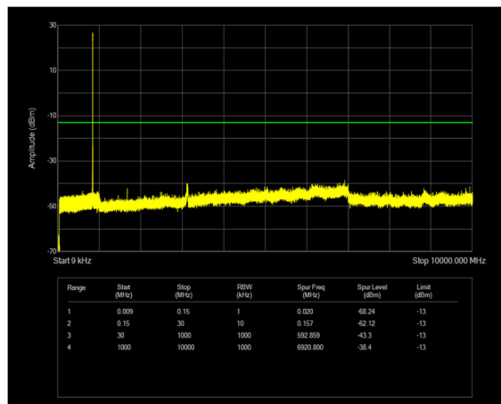
n26(824-849) SCS=15kHz DFT_QPSK BW=5MHz Channel=167300 RB=1@0
