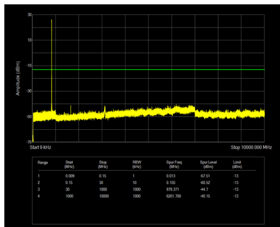
n26(824-849) SCS=15kHz DFT_QPSK BW=5MHz Channel=165300 RB=1@0
