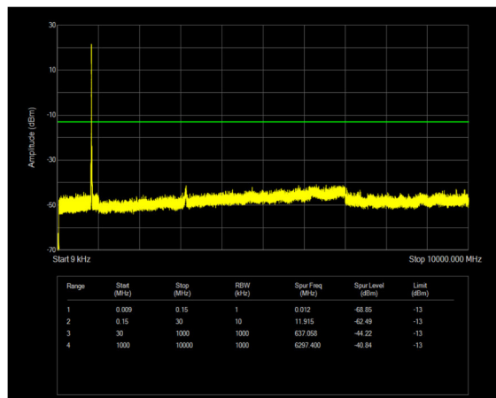
n26(824-849) SCS=15kHz DFT_QPSK BW=5MHz Channel=165300 RB=25@0
