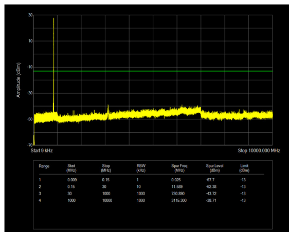
n26(824-849) SCS=15kHz DFT_QPSK BW=20MHz Channel=167800 RB=1@105
