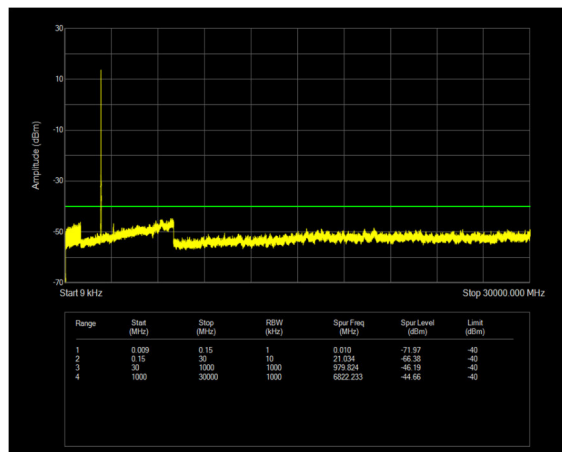
n30 SCS=15kHz CP_QPSK BW=10MHz Channel=462000 RB=52@0
