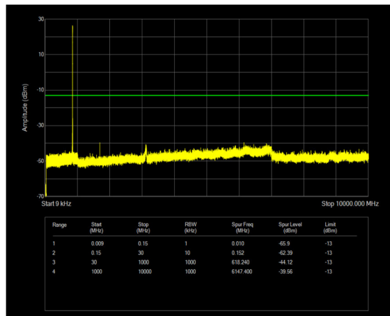
n26(824-849) SCS=15kHz DFT_QPSK BW=5MHz Channel=169300 RB=1@0
