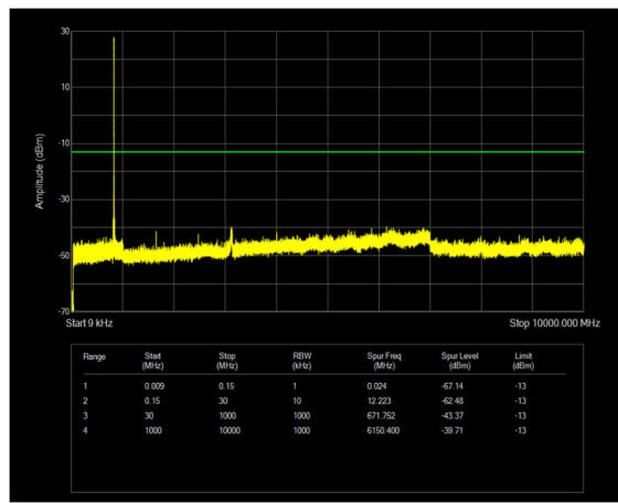
n26(824-849) SCS=15kHz DFT_QPSK BW=20MHz Channel=166800 RB=1@0
