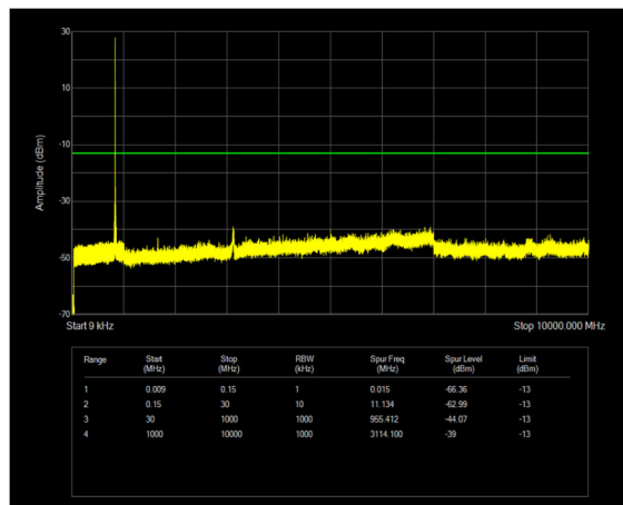
n26(824-849) SCS=15kHz DFT_QPSK BW=20MHz Channel=167800 RB=1@0
