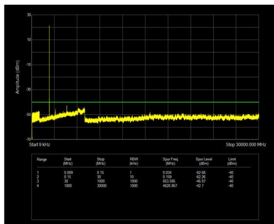
n30 SCS=15kHz CP_QPSK BW=10MHz Channel=462000 RB=1@51
