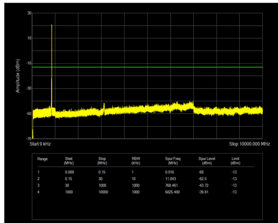
n26(824-849) SCS=15kHz DFT_QPSK BW=5MHz Channel=169300 RB=25@0
