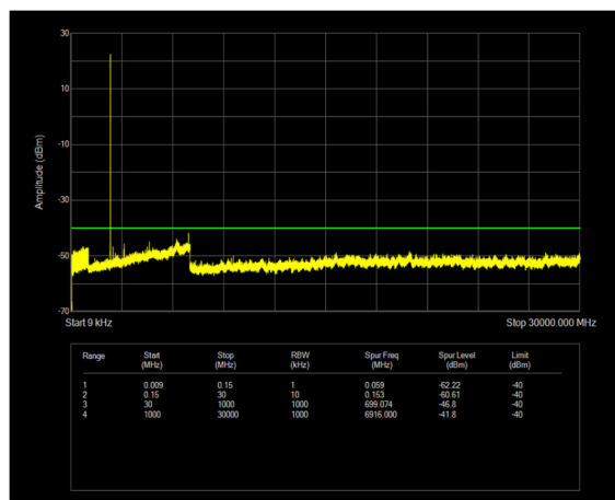
n30 SCS=15kHz CP_QPSK BW=10MHz Channel=462000 RB=1@0
