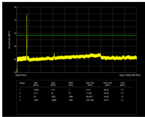
n26(824-849) SCS=15kHz DFT_QPSK BW=20MHz Channel=166800 RB=100@0
