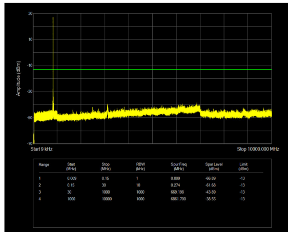
n26(824-849) SCS=15kHz DFT_QPSK BW=20MHz Channel=167300 RB=1@0
