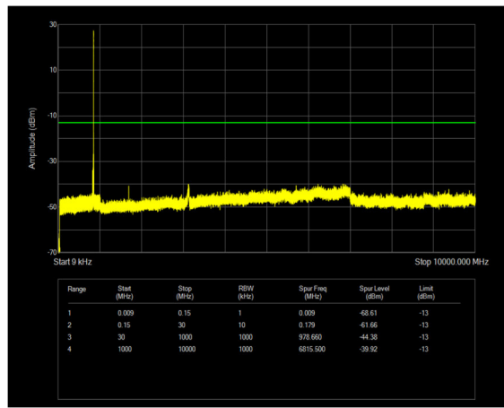
n26(824-849) SCS=15kHz DFT_QPSK BW=20MHz Channel=166800 RB=1@105
