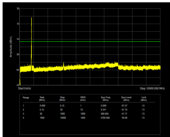
n26(824-849) SCS=15kHz DFT_QPSK BW=20MHz Channel=167800 RB=100@0
